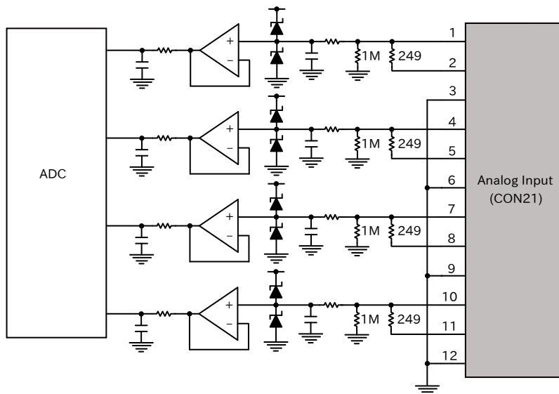
図 3.135 CON21 アナログ入力周辺回路
