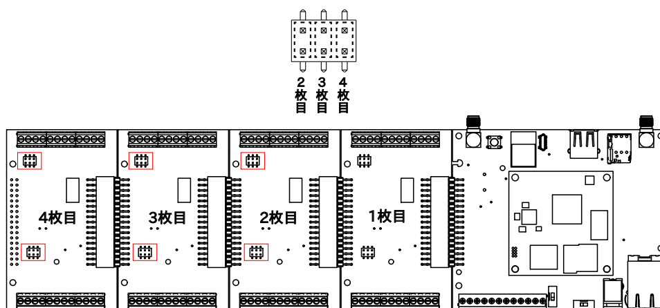
図 3.154 ピンヘッダの位置と設定
