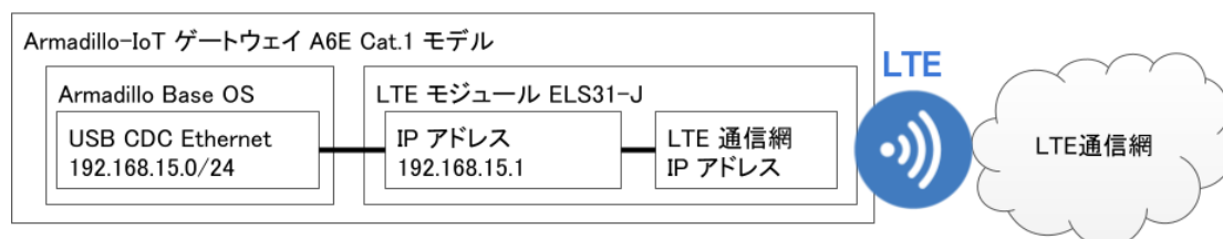
図 6.140 Cat.1 モデル (ELS31-J) LTE ネットワーク構成
