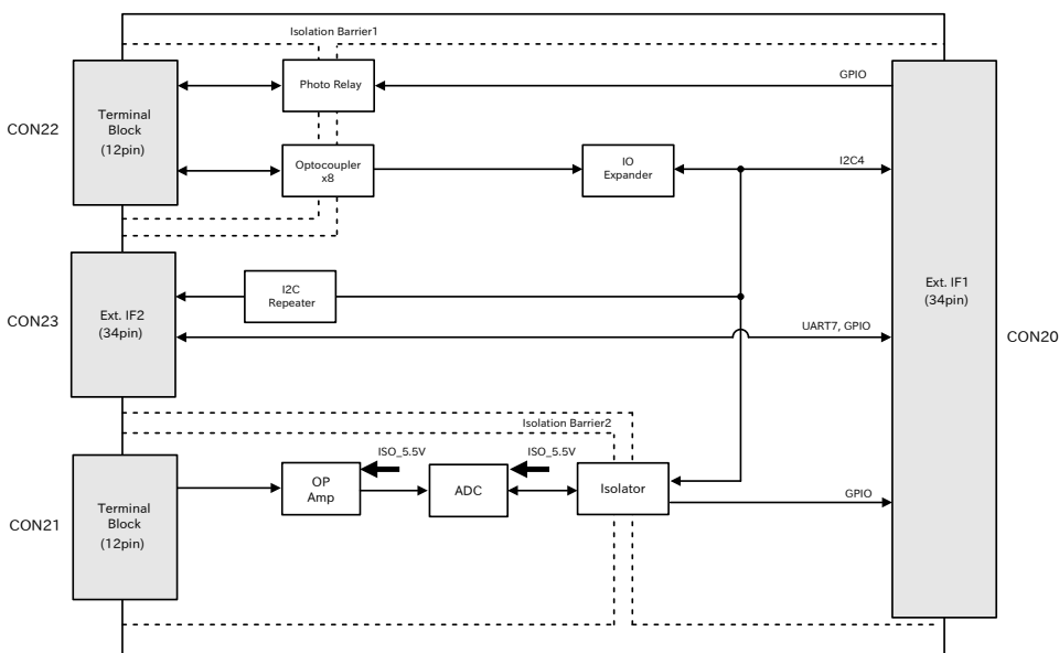
図 6.244 +Di8+Ai4 拡張基板のブロック図
