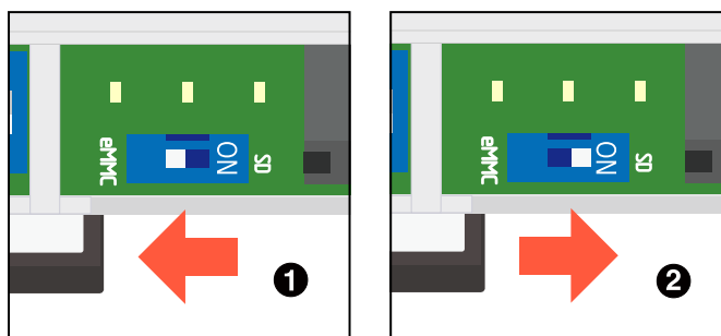
図 3.122 スイッチの状態と起動デバイス
