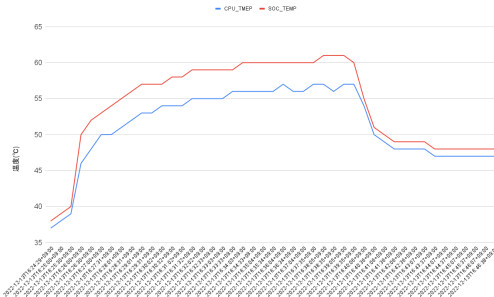
図 6.194 Armadillo-IoT ゲートウェイ G4 で取得した温度のグラフ
