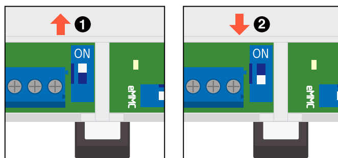
図 3.101 スwitchの状態と終端抵抗の ON/OFF
