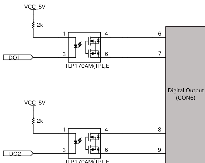
図 3.95 CON6 接点出力周辺回路
