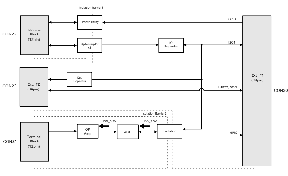
図 6.226 +Di8+Ai4 拡張基板のブロック図
