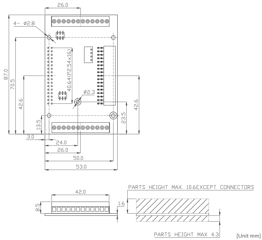
図 6.228 +Di8+Ai4 拡張基板基板形状図
