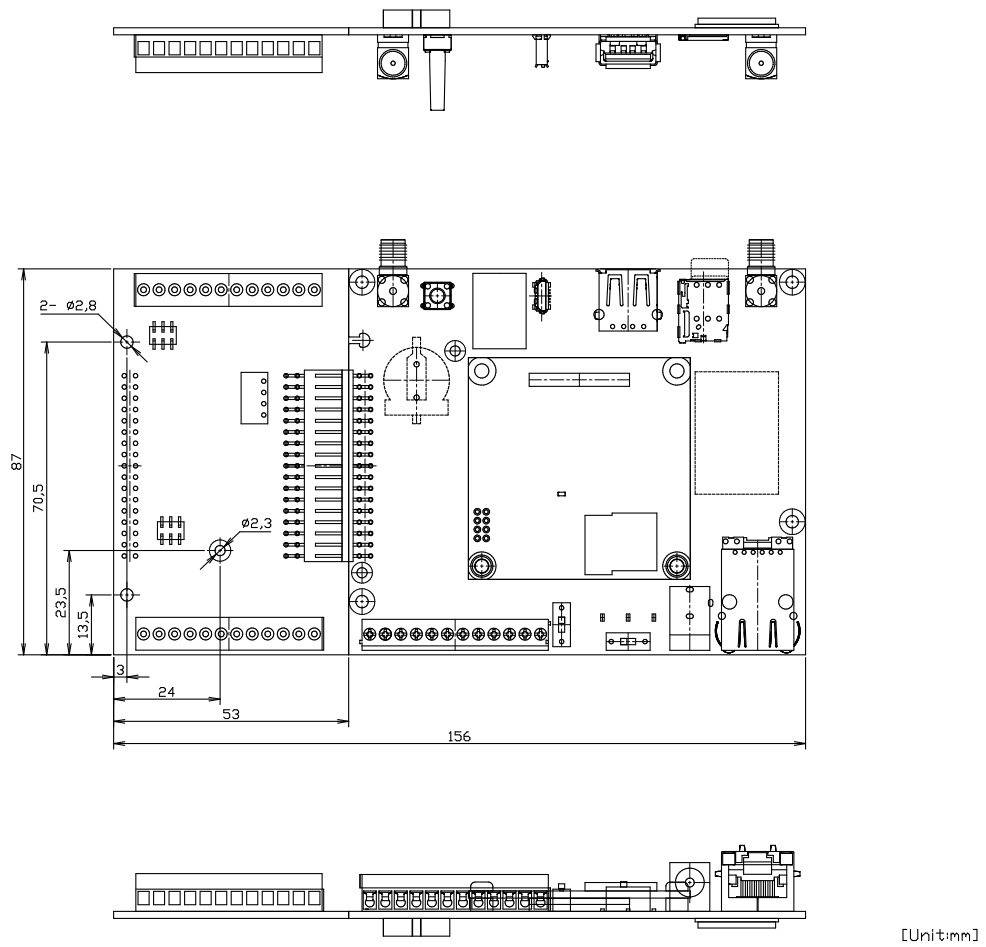
図 3.50 基板形状および固定穴寸法 2
