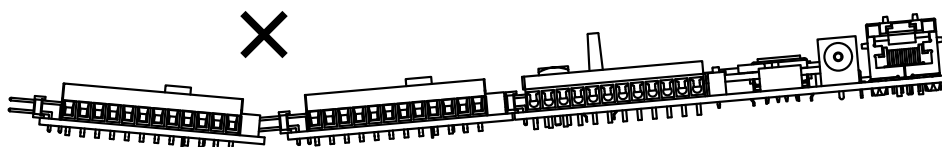
図 3.119 悪い組付け例
