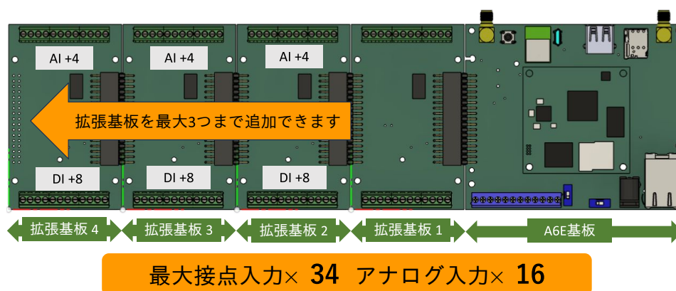
図 3.117 +Di8+Ai4 拡張基板のカスケード接続
