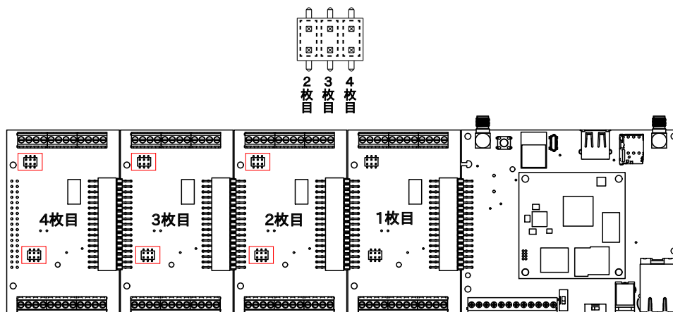
図 3.120 ピンヘッダの位置と設定
