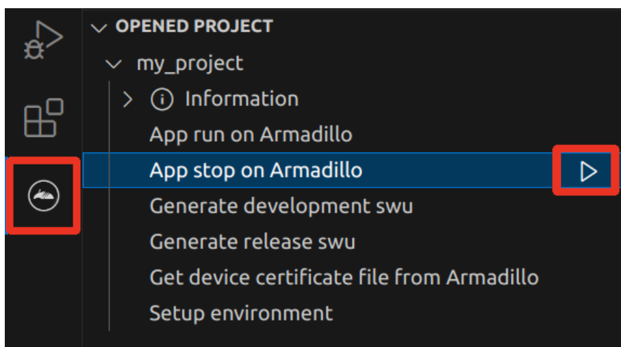
図 3.168 ゲートウェイコンテナアプリケーションを終了する
