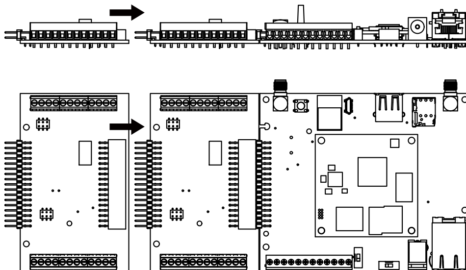
図 3.118 +Di8+Ai4 拡張基板の組付け方法
