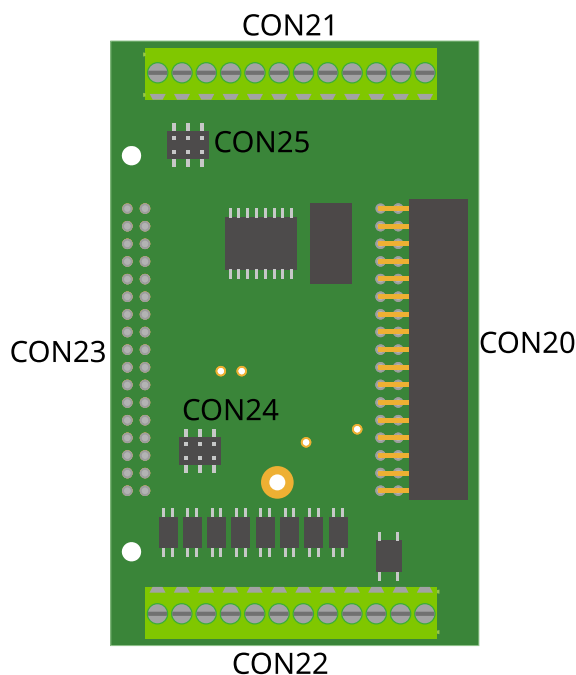
図 6.214 +Di8+Ai4 拡張基板のインターフェースレイアウト
