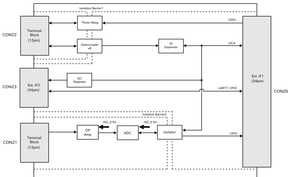
図 6.213 +Di8+Ai4 拡張基板のブロック図
