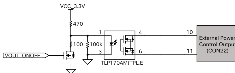
図 3.113 CON22 外部電源制御出力周辺回路
