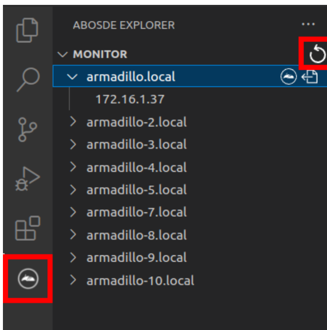
図 3.129 ABOSDE に表示されている Armadillo を更新する
