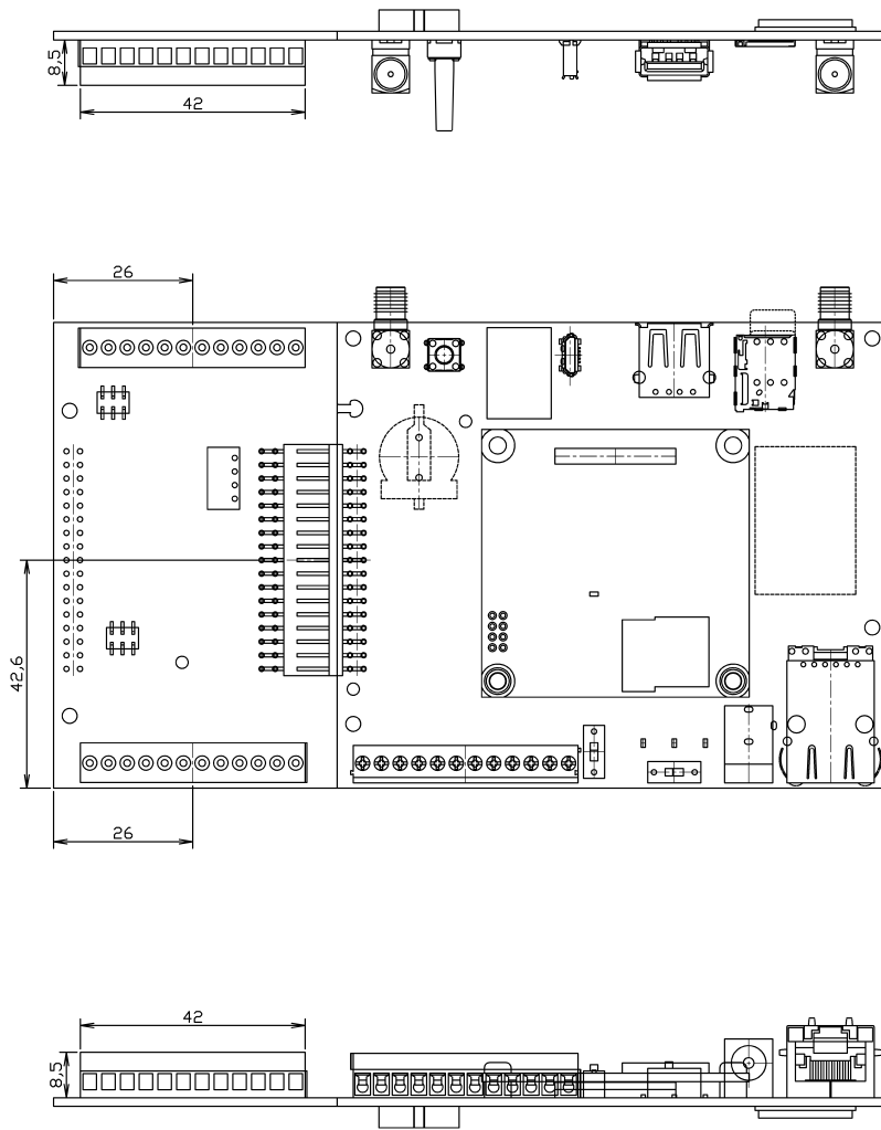
図 6.196 コネクタ中心寸法 2
