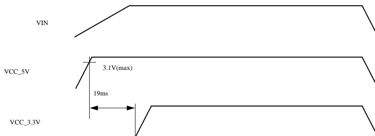
図 6.191 電源シーケンス
