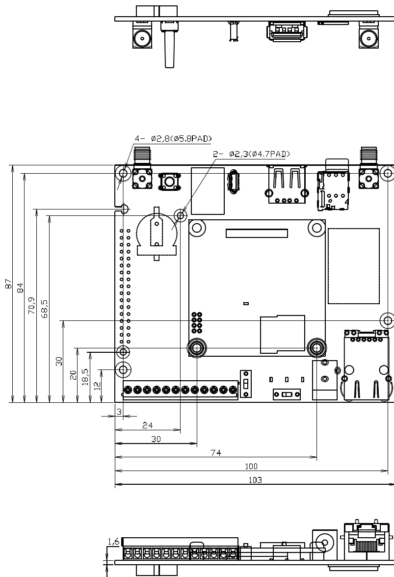
図 6.193 基板形状および固定穴寸法 1
