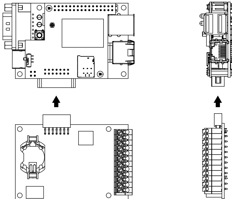
図 20.10 組み立て図
