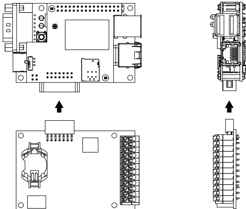
図 20.10 組み立て図
