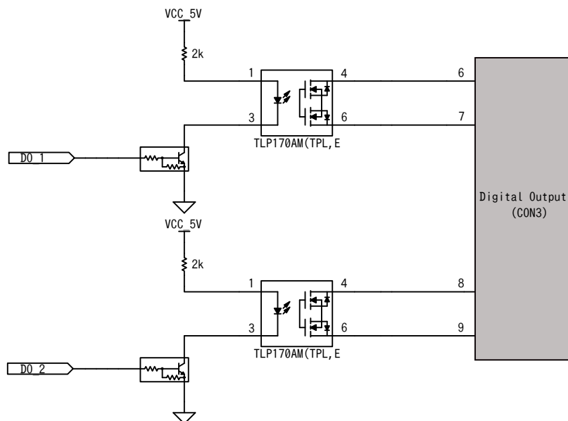
図 20.8 CON3 デジタル出力部
