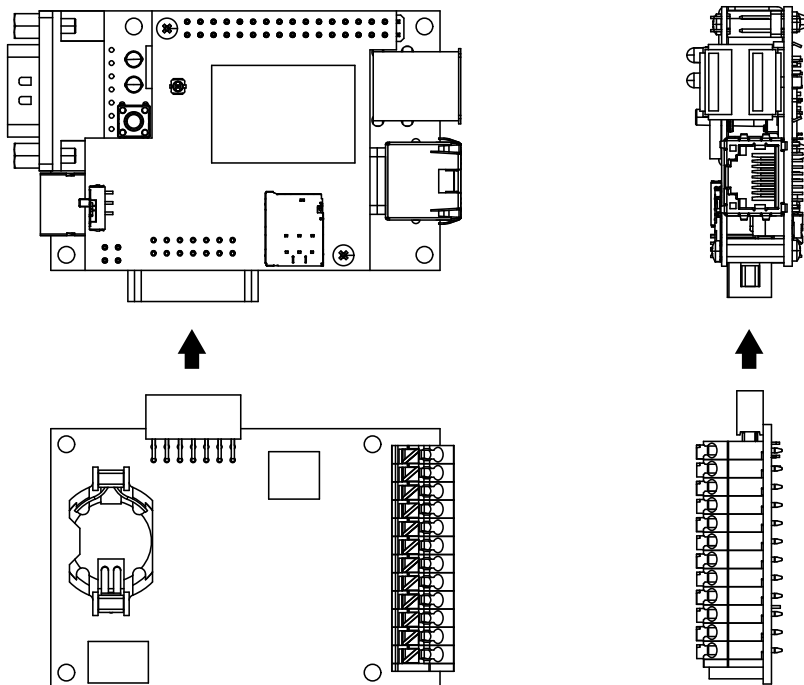
図 20.10 組み立て図
