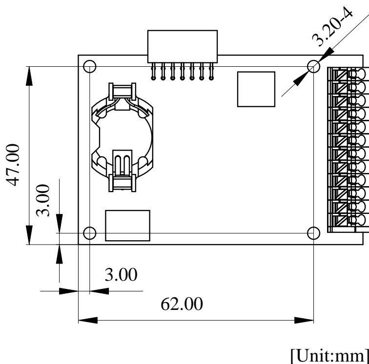
図 20.13 固定穴寸法
