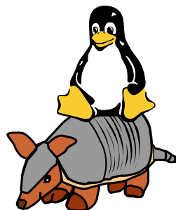
図 3.1 Armadillo ロゴ
