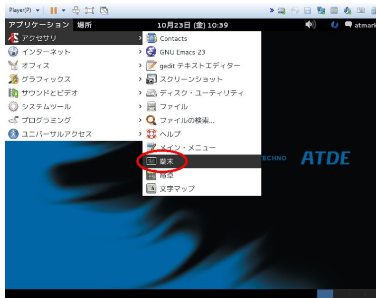
図 6.19 端末の起動
