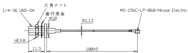
図 17.2 アンテナ形状
