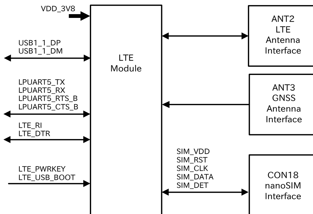
図 5.92 LTE インターフェース回路構成
