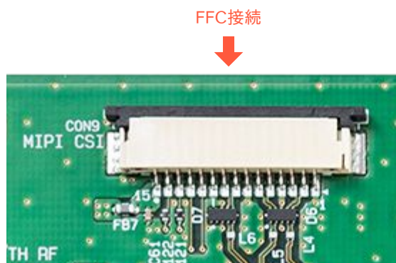
図 5.115 MIPI CSI FFC 接続
