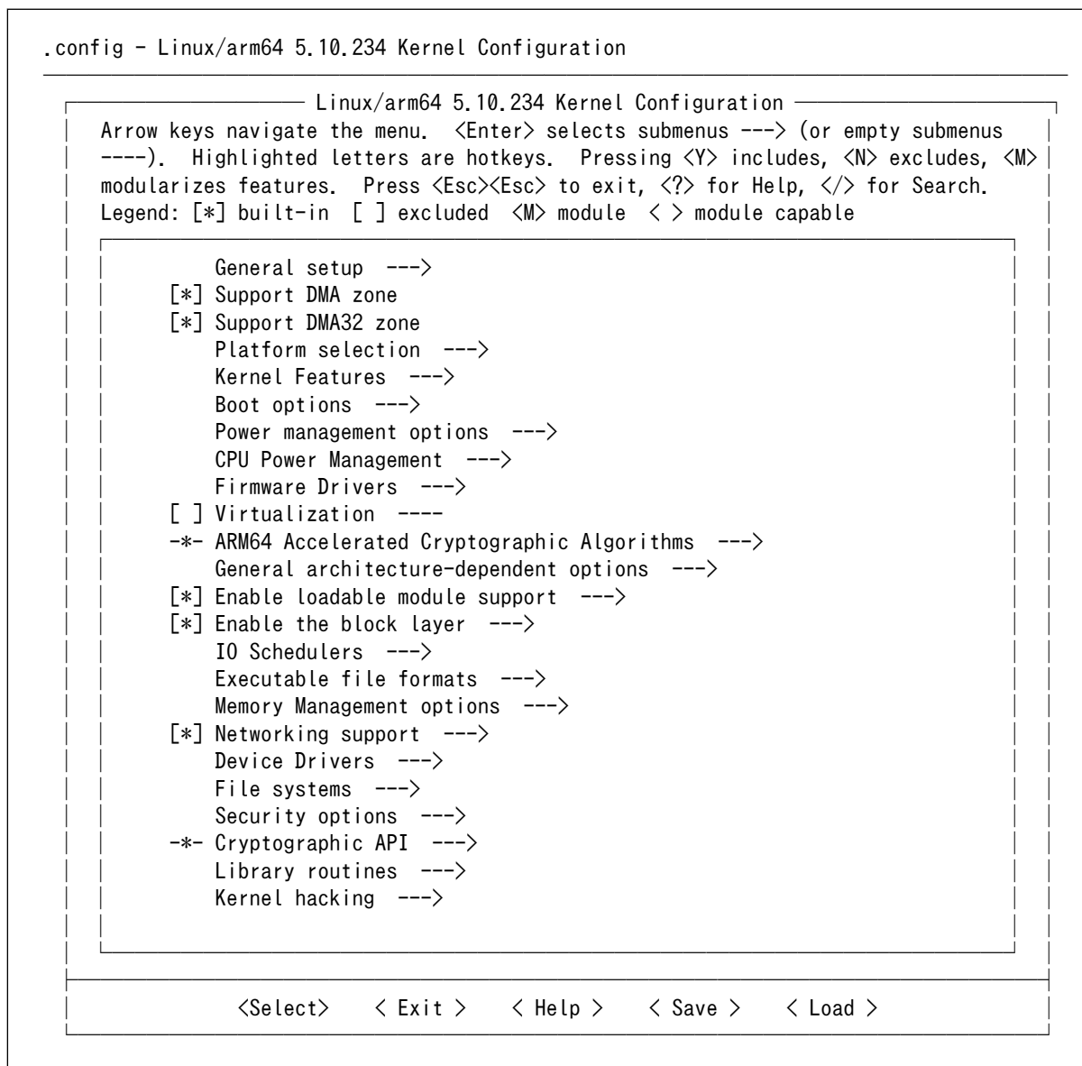
図 10.88 Linux カーネルコンフィギュレーション設定画面
