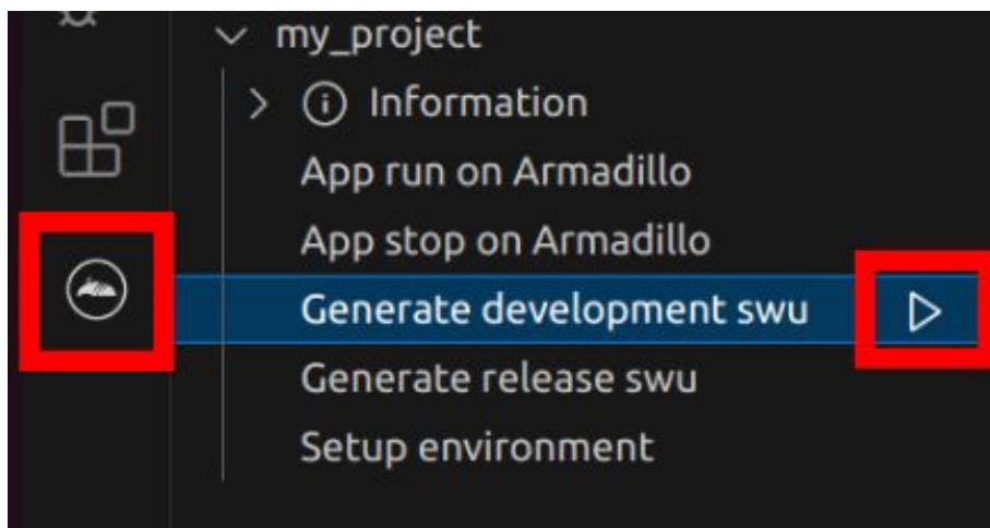
図 7.144 VS Code でコンテナイメージの作成を行う
