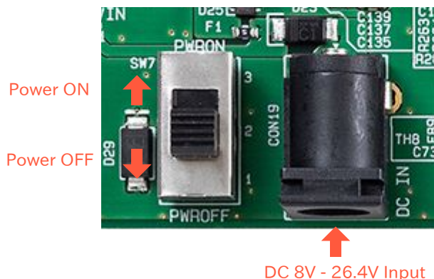
図 5.73 電源入力
