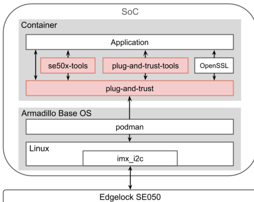
図 10.119 Plug & Trust Middleware の周辺のソフトウェアスタック
