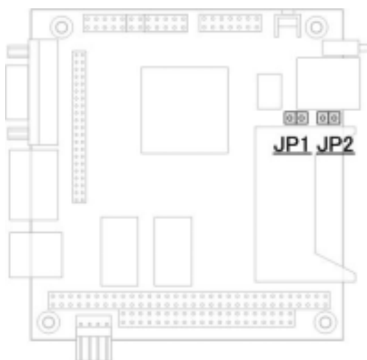
図 2-2 ジャンパの位置
