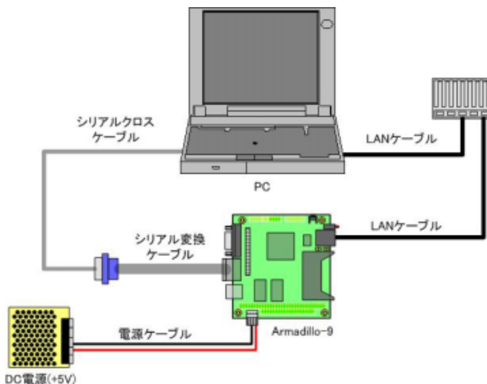
図 2-1 Armadillo-9 接続例
