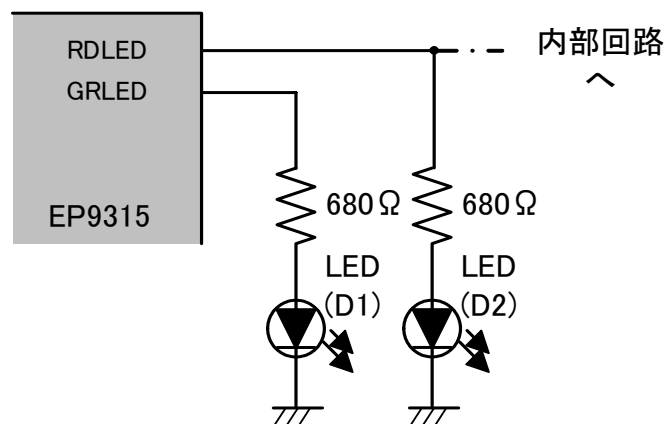
図 6-3 LED(D1)の接続
