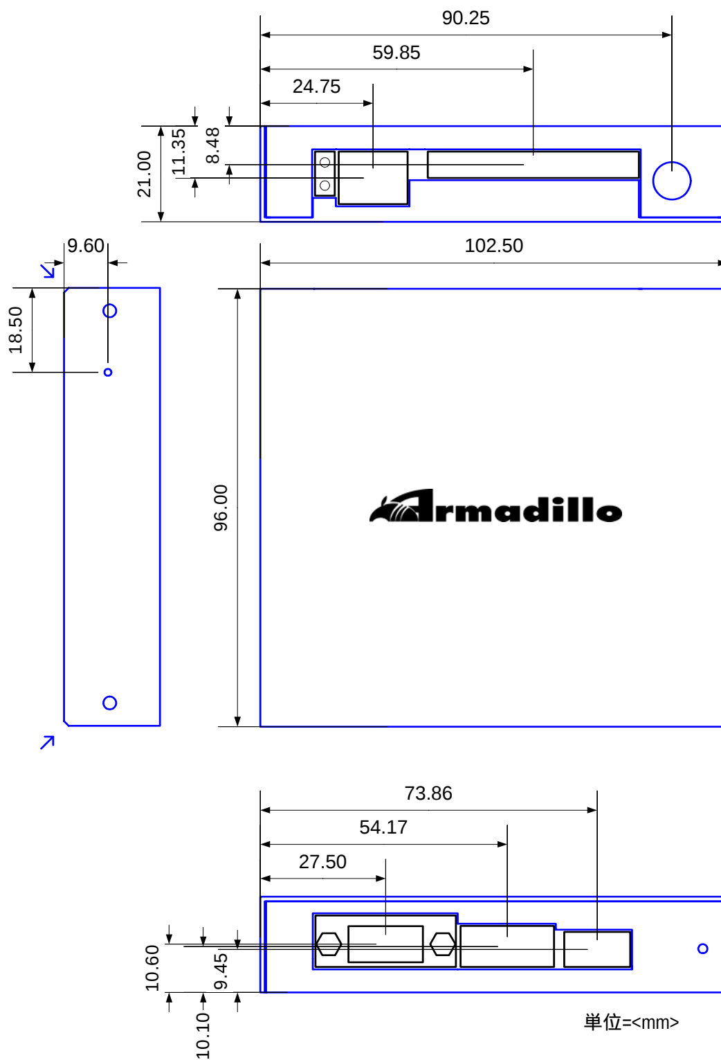
Armadillo-9 ケースモデル形状図
