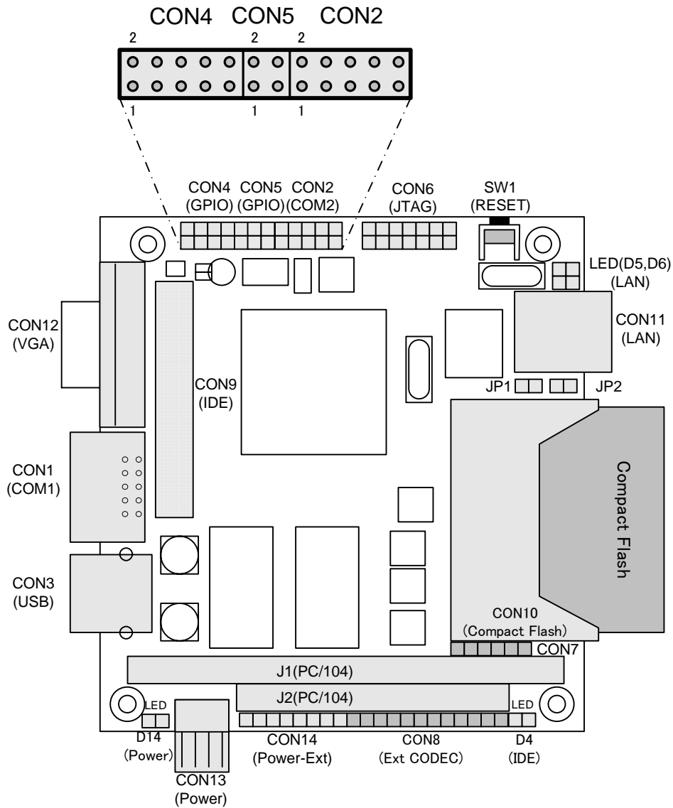
図 2-1 見取り図
