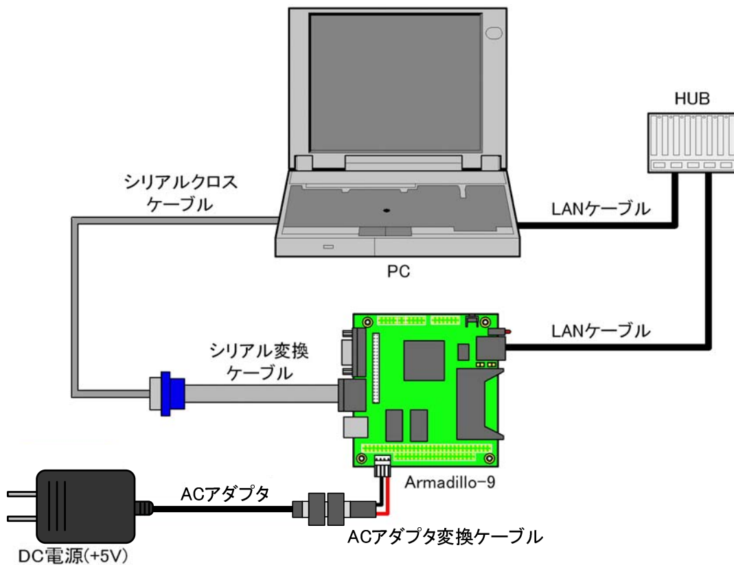
図 2-2 接続図
