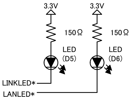
図 5-6 LED(D5,6)の接続
