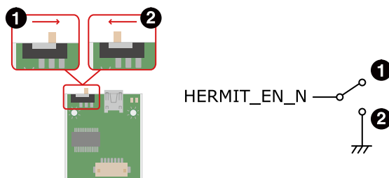
図 20.8 スライドスイッチについて
