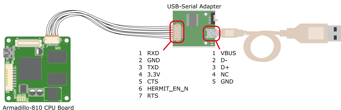
図 20.7 開発用 USB シリアル変換アダタの配線
