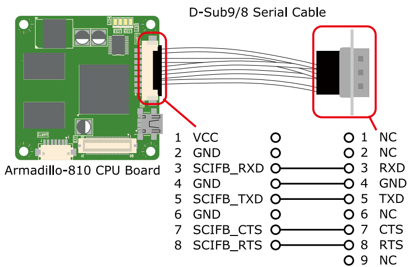
図 20.9 D-Sub9/8 ピン シリアル変換ケーブルの配線
