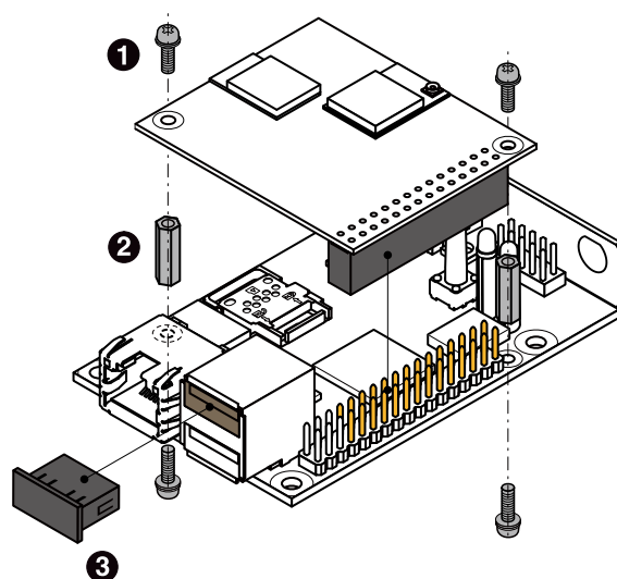
図 6.199 WLAN コンボ、BT/TH オプションモジュールの組み立て
