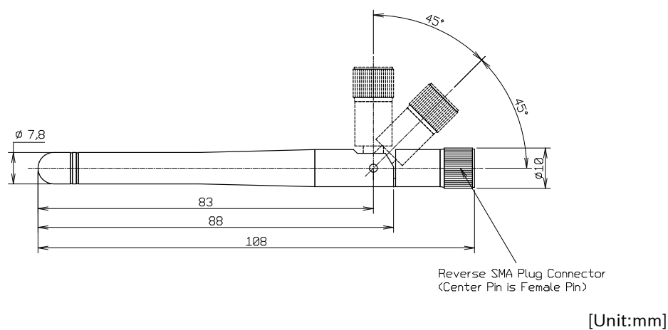
図 6.211 無線 LAN 用 外付けアンテナ 08 形状図
