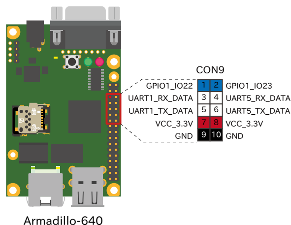
図 6.182 Armadillo-640 のシリアル信号線
