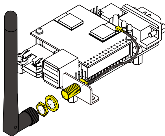
図 6.217 アンテナ固定金具へのアンテナの固定
