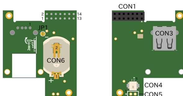
図 6.189 RTC オプションモジュールのインターフェース
