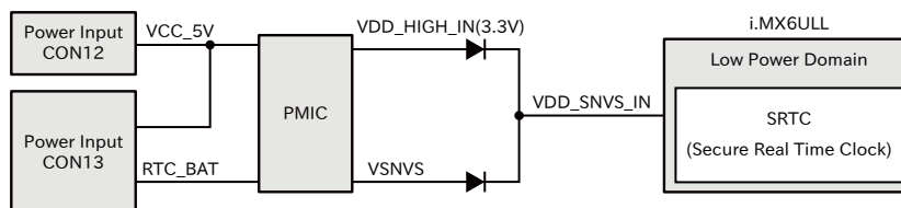
図 3.125 バックアップ電源供給
