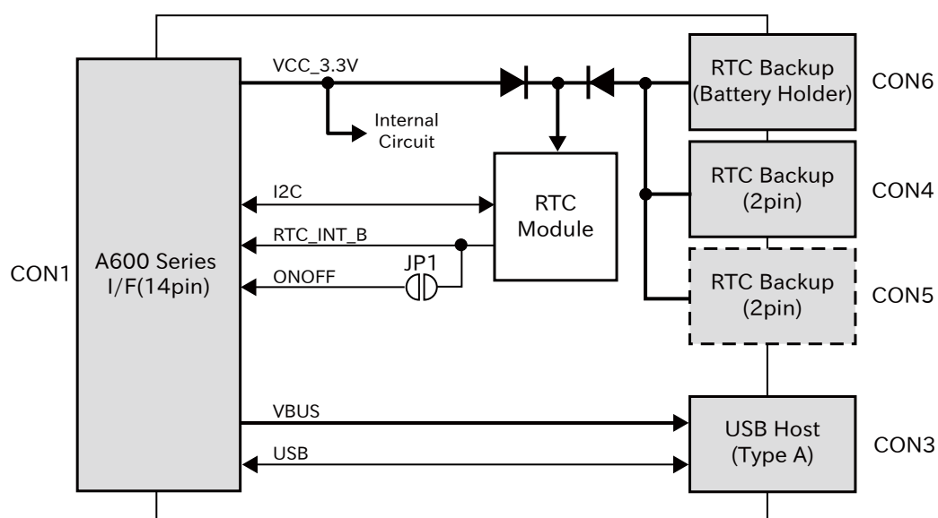
図 6.188 RTC オプションモジュールのブロック図
