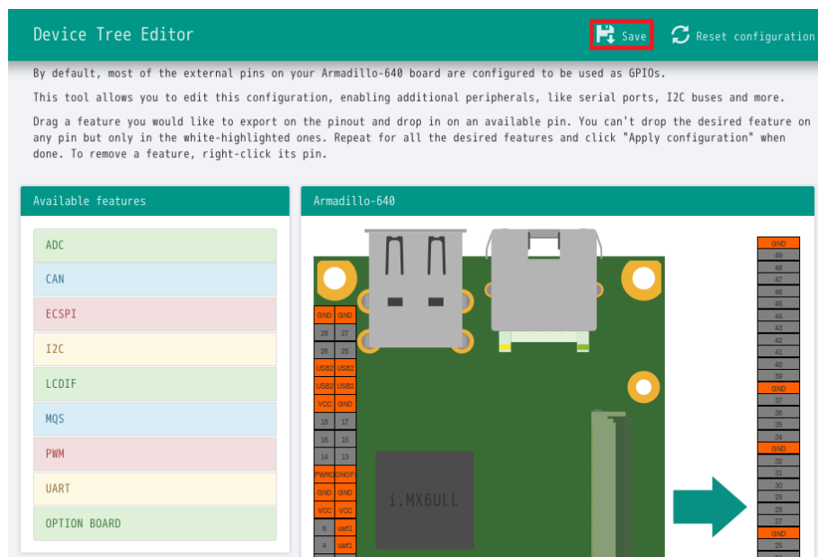
図 3.74 DTS/DTB の生成
