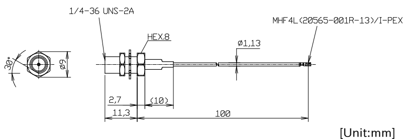
図 6.212 無線 LAN 用 外付けアンテナケーブル 08 形状図
