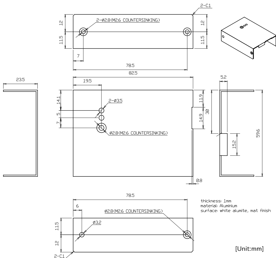
図 6.186 金属ケース(上板)寸法図
