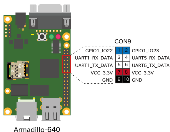
図 6.176 Armadillo-640 のシリアル信号線
