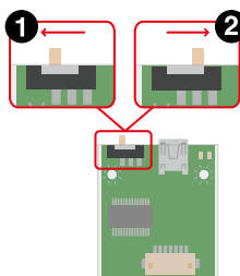
図 3.47 スライドスイッチの設定
