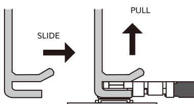
図 6.204 挿抜治具によるアンテナケーブルコネクタの抜去
