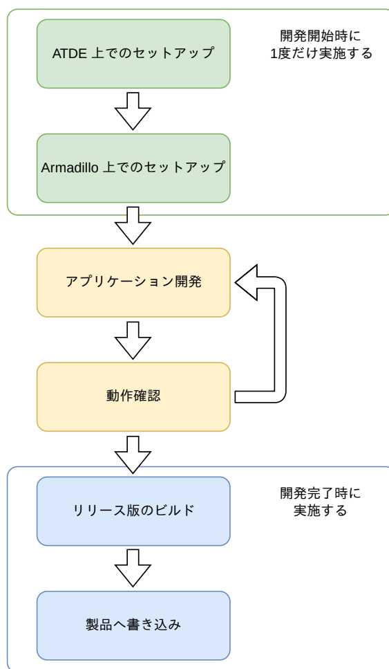
図 3.164 CUI アプリケーション開発の流れ
