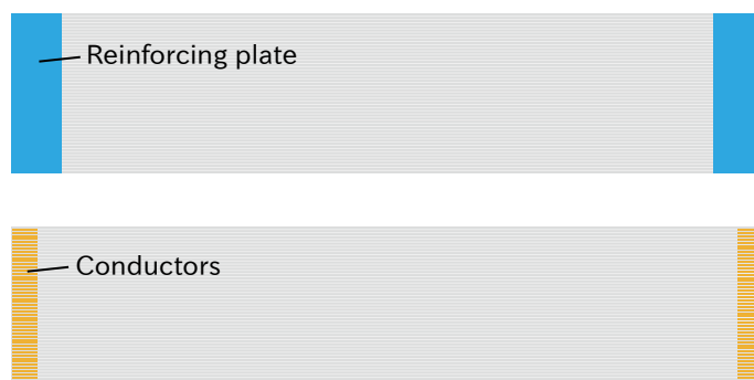
図 3.123 フレキシブルフラットケーブルの形状
