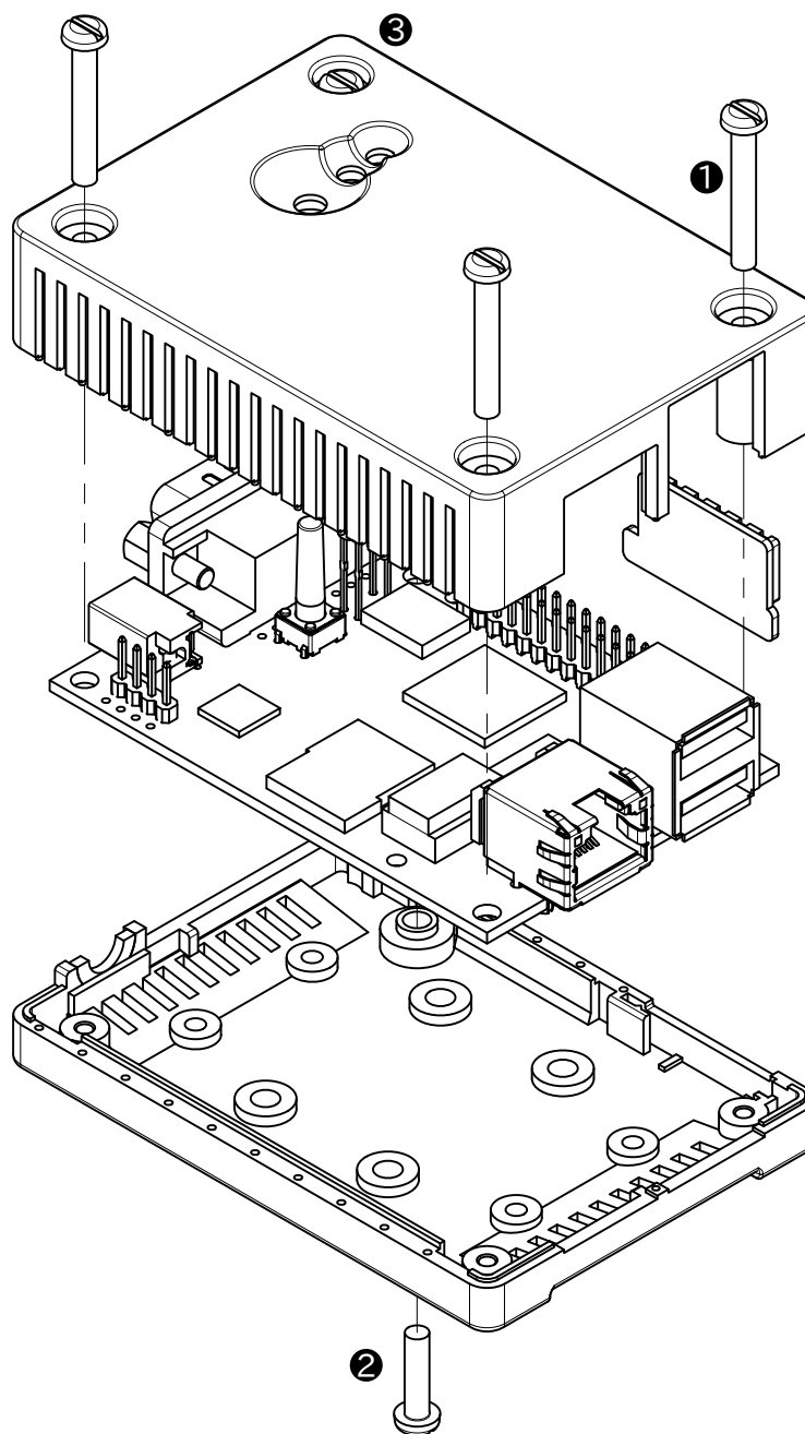
図 6.177 Armadillo-600 シリーズ オプションケース(樹脂製)の組み立て
