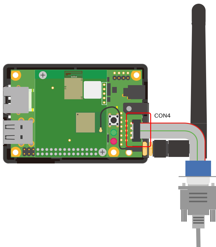
図 6.198 CON4 をシリアルコンソールとして使用する場合の接続例
