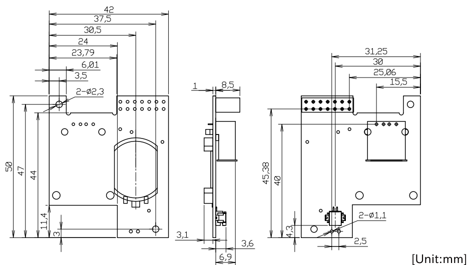
図 6.188 RTC オプションモジュール形状
