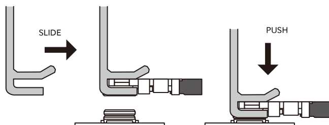
図 6.201 挿抜治具によるアンテナケーブルコネクタの嵌合
