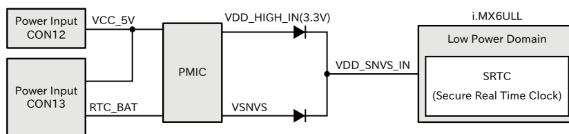
図 3.125 バックアップ電源供給
