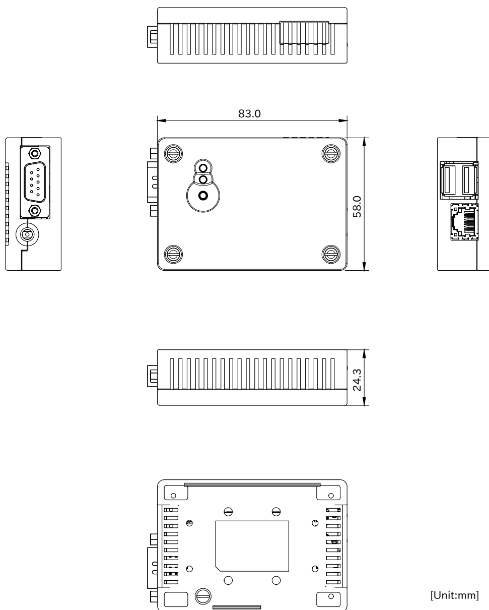
図 6.178 樹脂ケース形状図
