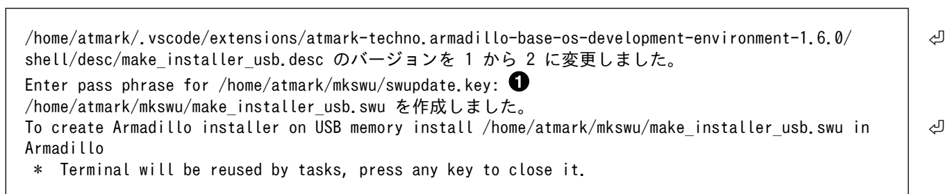
図 4.8 make-installer.swu 生成時のログ
