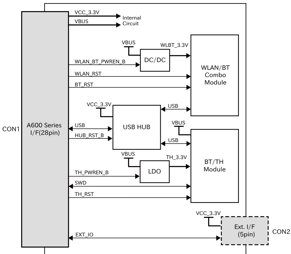
図 6.159 WLAN コンボ、BT/TH オプションモジュールのブロック図
