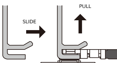
図 6.173 挿抜治具によるアンテナケーブルコネクタの抜去
