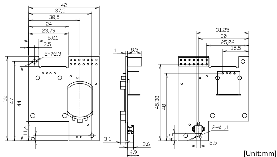
図 6.157 RTC オプションモジュール形状
