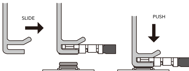
図 6.170 挿抜治具によるアンテナケーブルコネクタの嵌合
