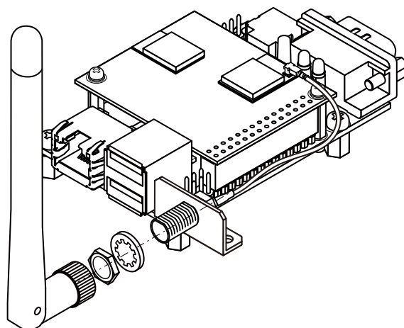
図 6.163 外付けアンテナの組み立て(OP-MNT-ANT-MET-00 使用)
