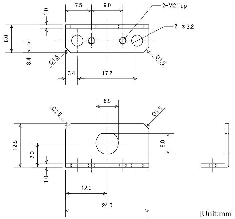
図 6.181 アンテナ固定金具 形状図
