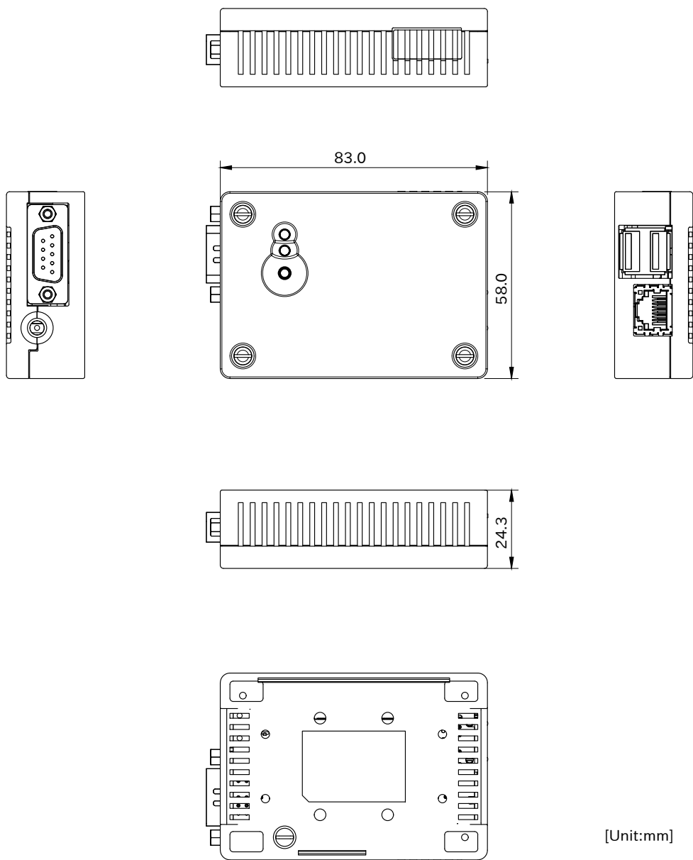
図 6.147 樹脂ケース形状図
