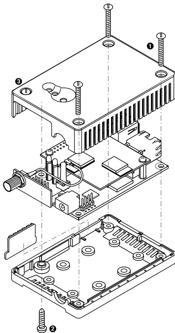
図 6.165 ケースの組み立て
