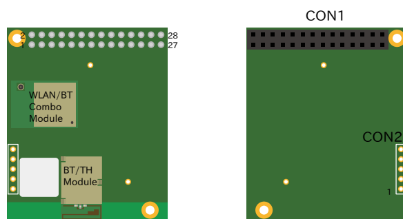
図 6.160 WLAN コンボ、BT/TH オプションモジュールのインターフェース
