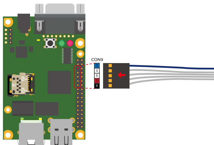
図 4.13 CON9-USB シリアル変換アダプタ接続図
