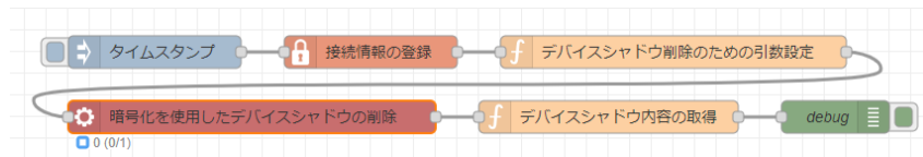
図 4.73 データの暗号化を使用したデバイスシャドウを削除するフロー
