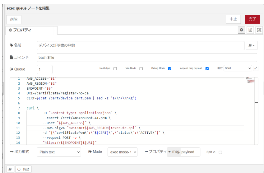
図 4.49 [デバイス証明書の登録] ノードのプロパティ内容
