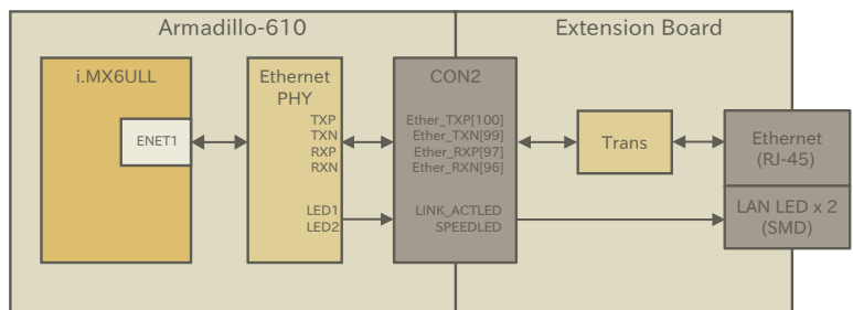
図 3.31 LAN(Ethernet)接続例
