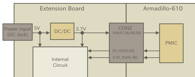
図 3.29 電源回路例
