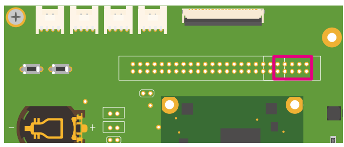
図 6.150 Armadillo-610 拡張ボード CON21
