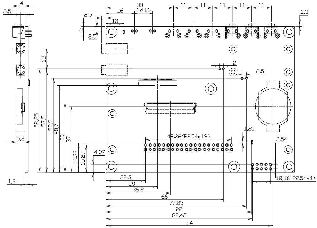
図 6.170 LCD 拡張ボードのコネクタ位置寸法
