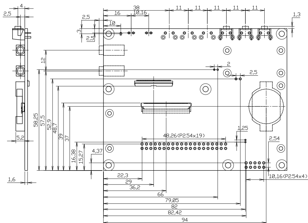
図 6.235 LCD 拡張ボードのコネクタ位置寸法
