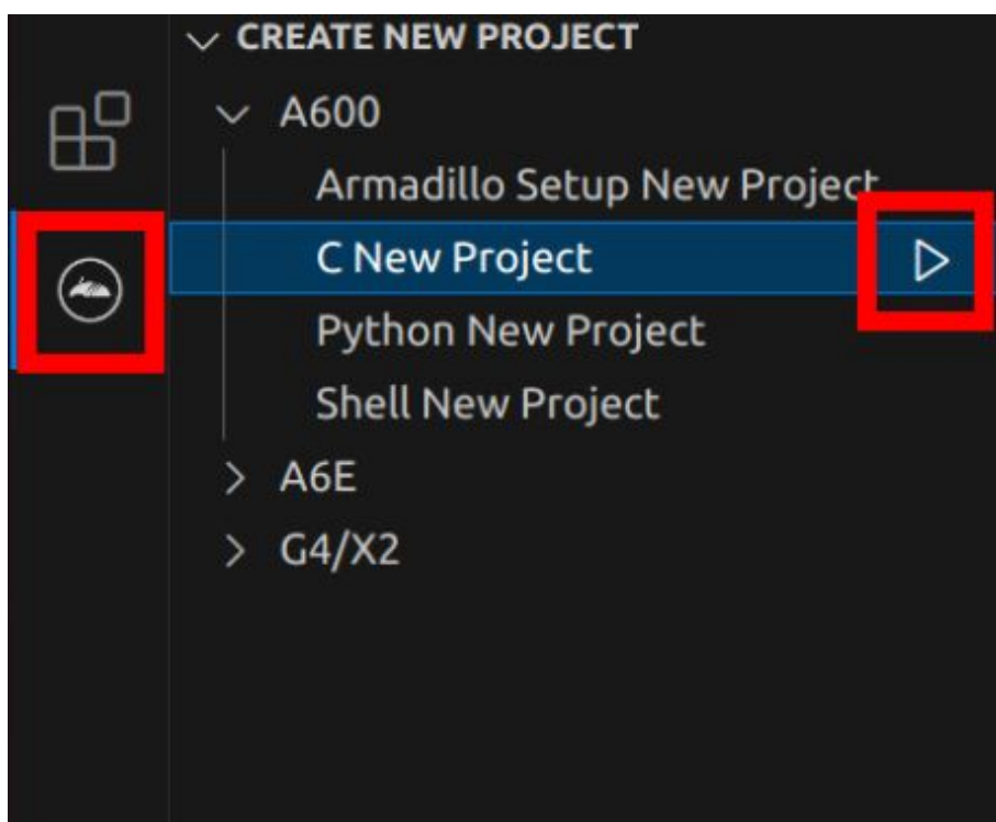
図 3.213 プロジェクトを作成する
