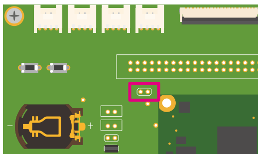
図 6.208 Armadillo-610 拡張ボード CON14
