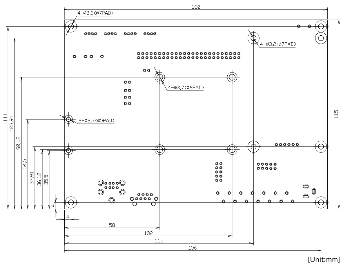
図 6.225 Armadillo-610 拡張ボード 基板形状および固定穴寸法
