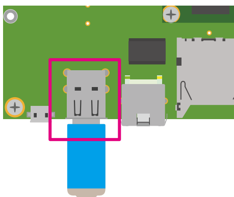
図 6.197 Armadillo-610 拡張ボード CON5
