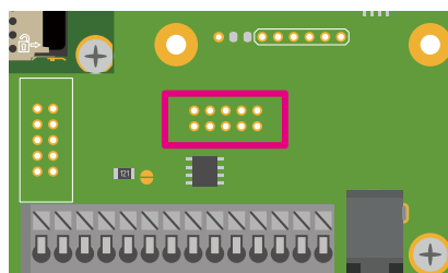
図 6.216 Armadillo-610 拡張ボード CON22
