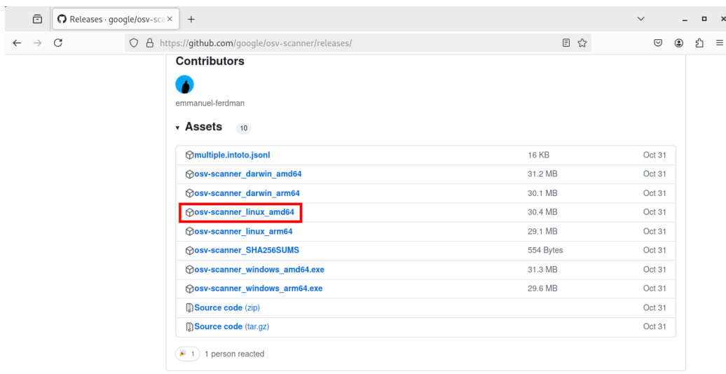
図 3.249 OSV-Scanner の実行ファイルをダウンロード
