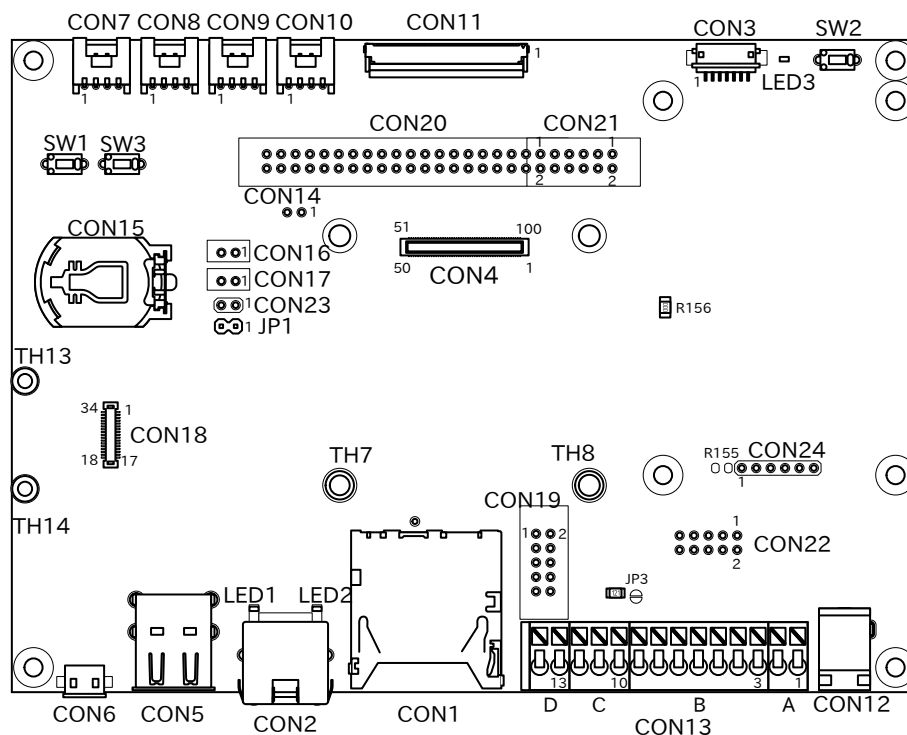
図 6.191 Armadillo-610 拡張ボードのインターフェースの概要
