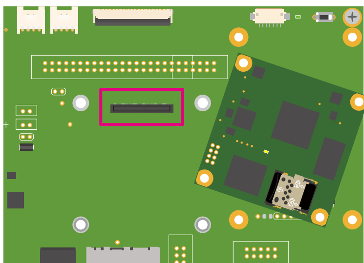
図 6.196 Armadillo-610 拡張ボード CON4
