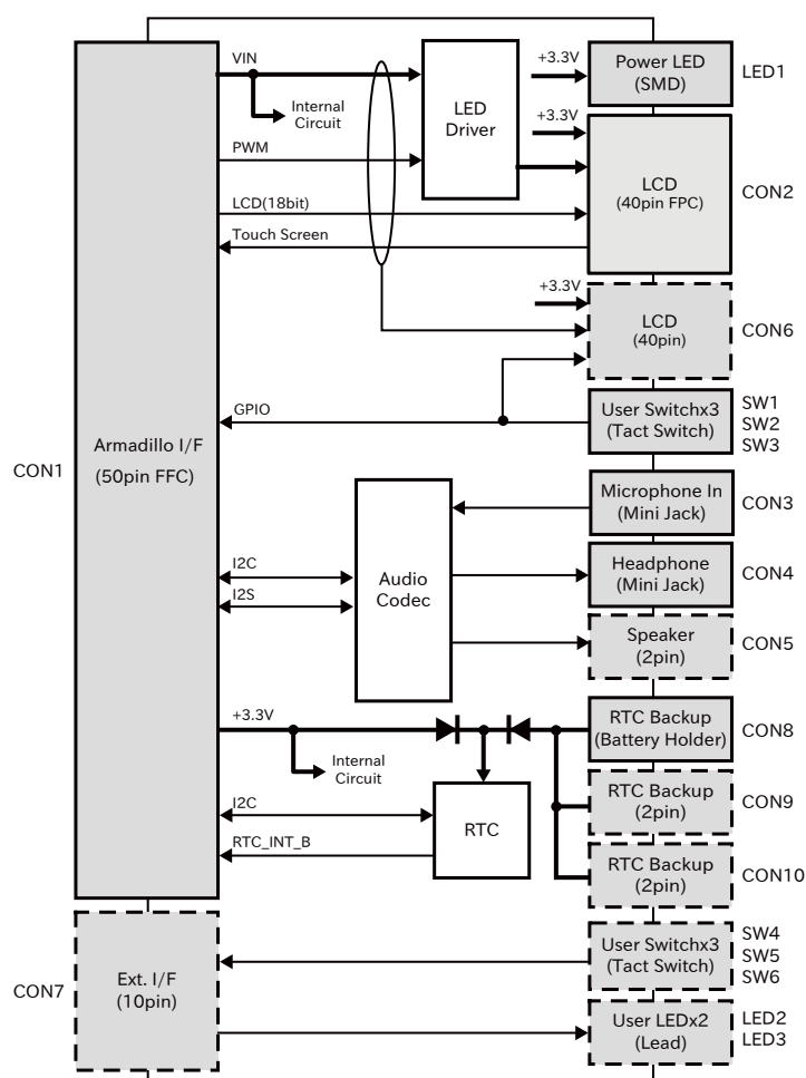
図 6.227 LCD 拡張ボードのブロック図
