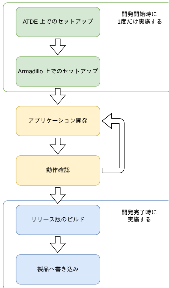
図 3.212 C 言語によるアプリケーション開発の流れ
