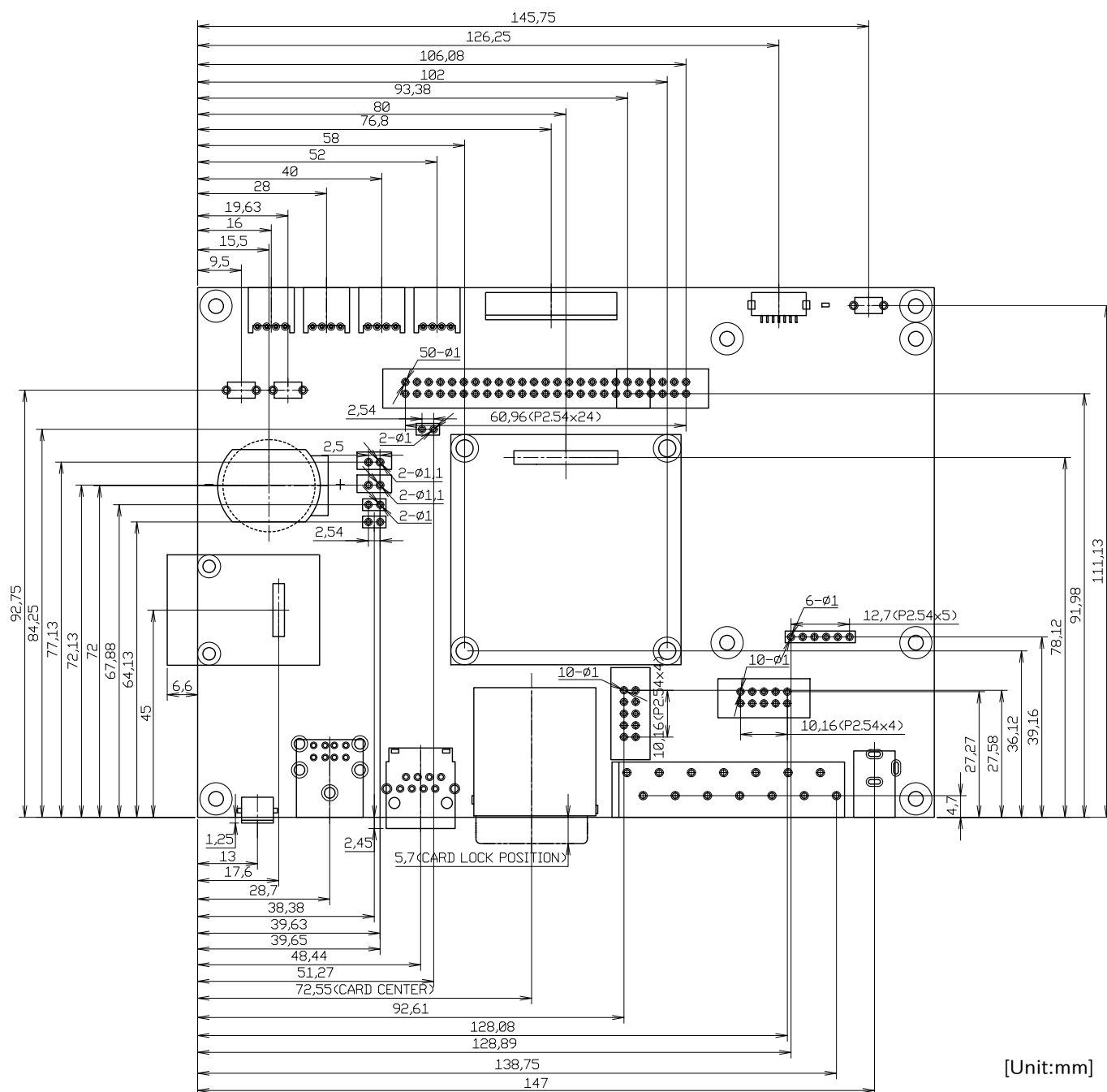
図 6.226 Armadillo-610 拡張ボード コネクタ中心寸法および穴寸法
