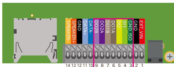
図 6.204 CON13B の配置
