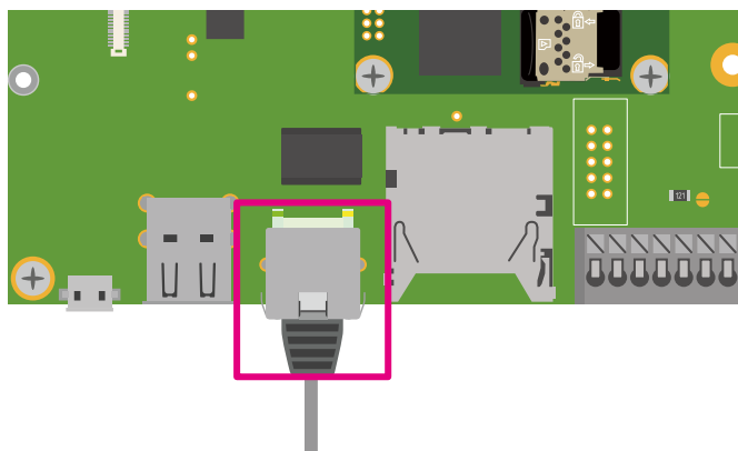
図 6.193 Armadillo-610 拡張ボード CON2
