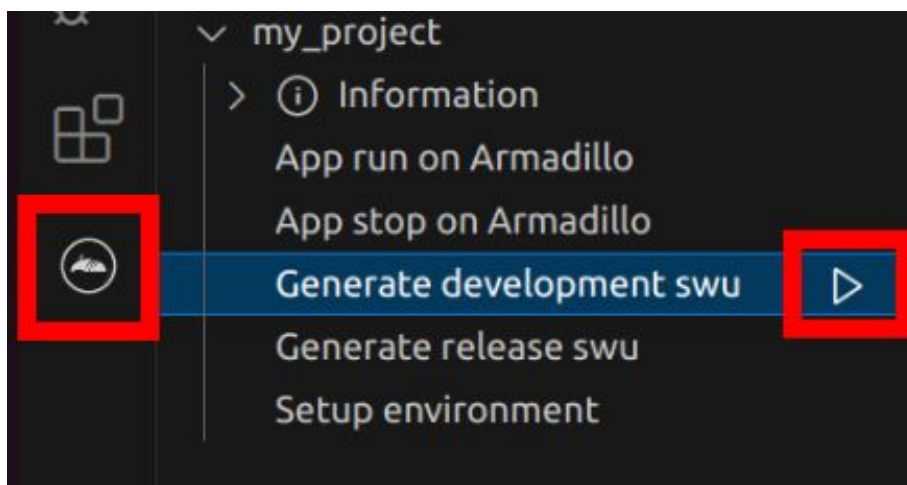
図 3.187 VS Code でコンテナイメージの作成を行う
