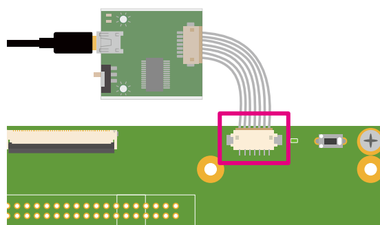
図 6.195 Armadillo-610 拡張ボード CON3
