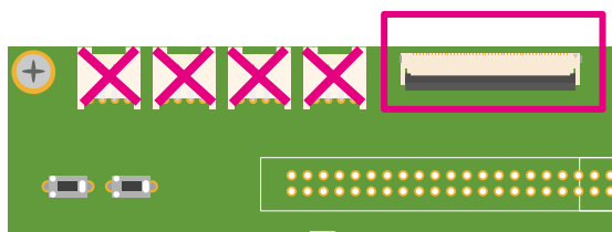
図 6.200 Armadillo-610 拡張ボード CON11
