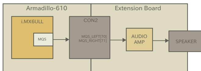
図 3.68 MQS 接続例
