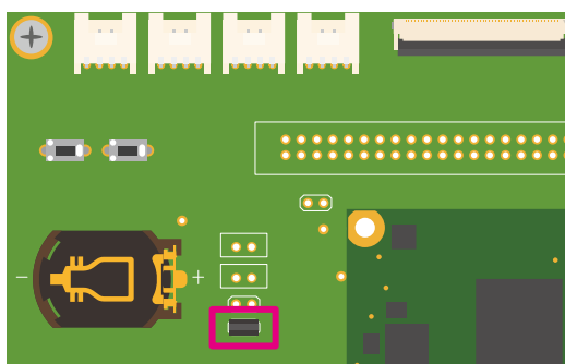
図 6.219 Armadillo-610 拡張ボード JP1
