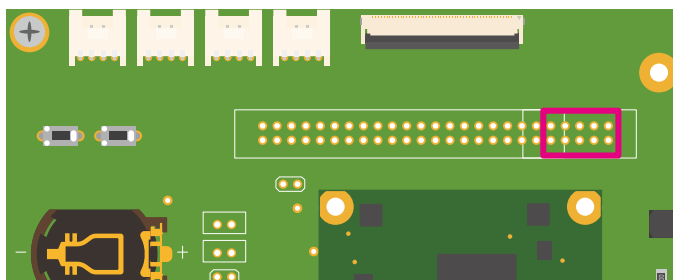
図 6.215 Armadillo-610 拡張ボード CON21
