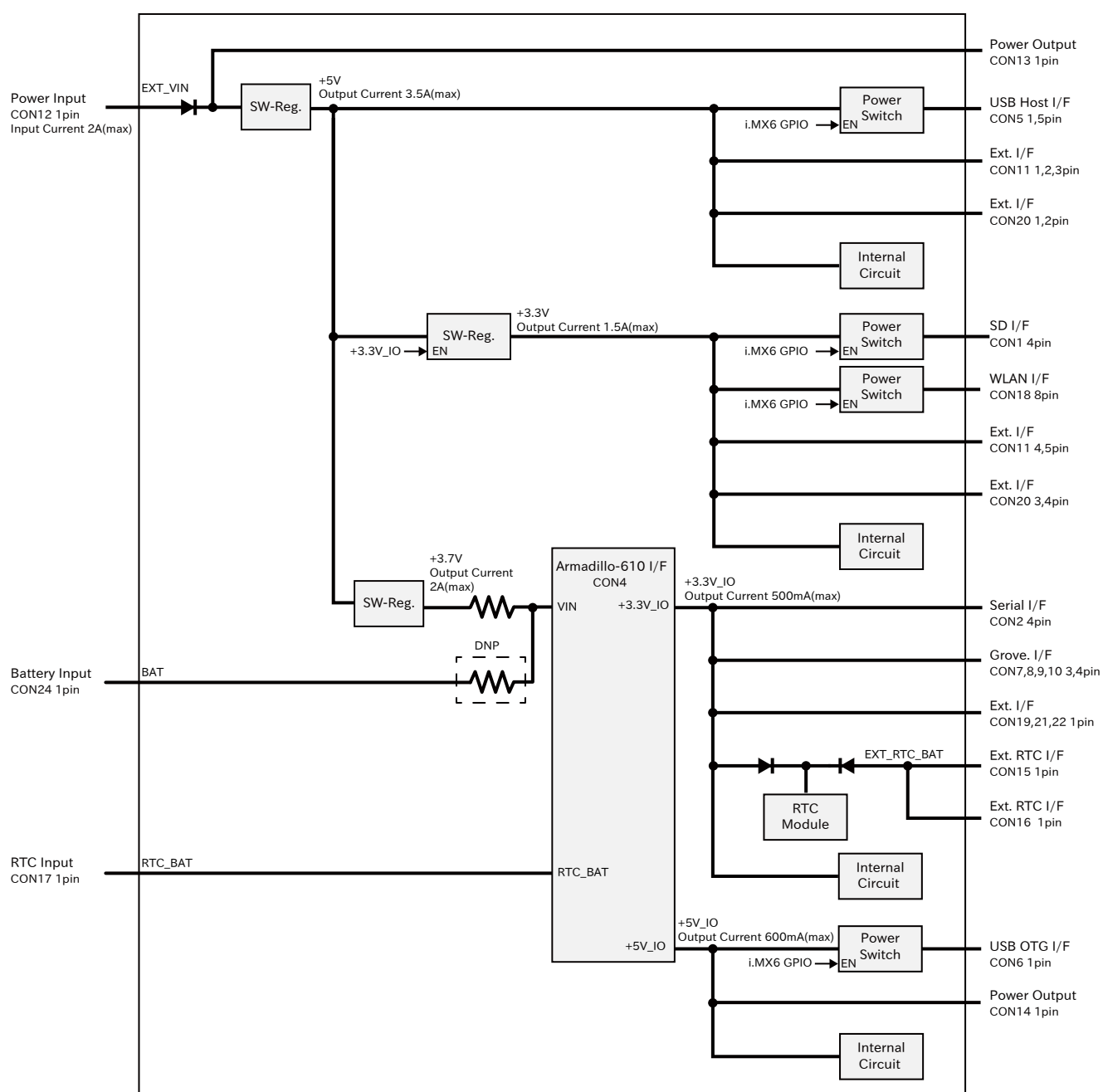
図 6.183 Armadillo-610 拡張ボードの電源回路の構成
