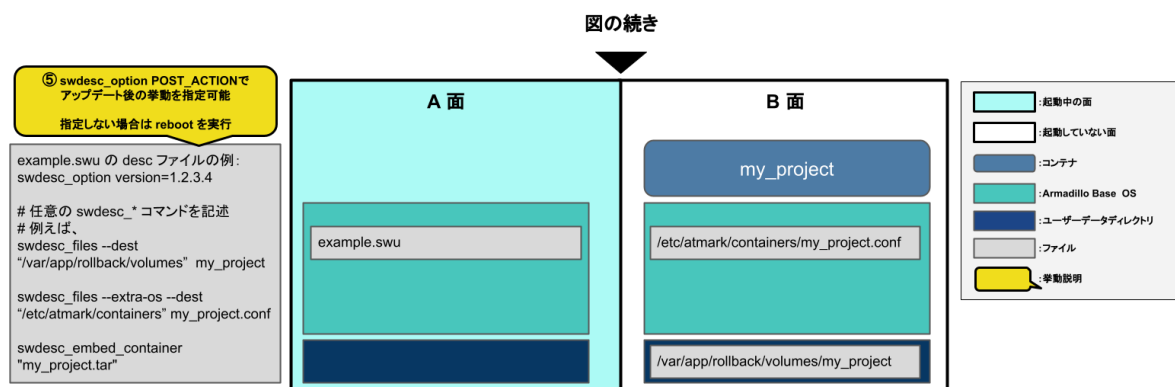
図 6.81 アップデート完了後の挙動
