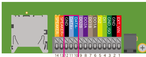
図 6.198 CON13C の配置
