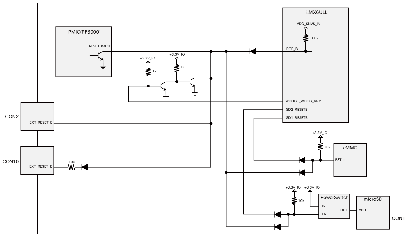
図 3.75 リセット回路の構成
