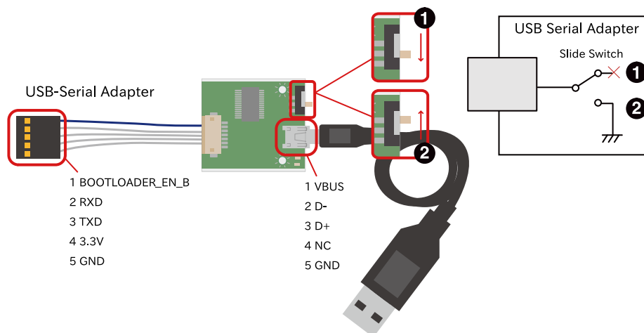
図 6.181 USB シリアル変換アダプタの配線
