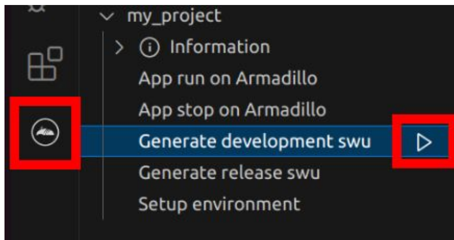
図 3.219 VS Code でコンテナイメージの作成を行う
