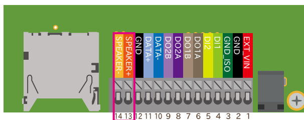
図 6.200 CON13D の配置
