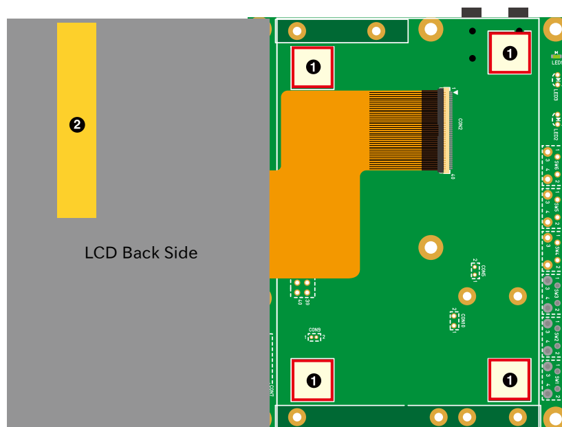
図 6.223 両面テープの貼付位置
