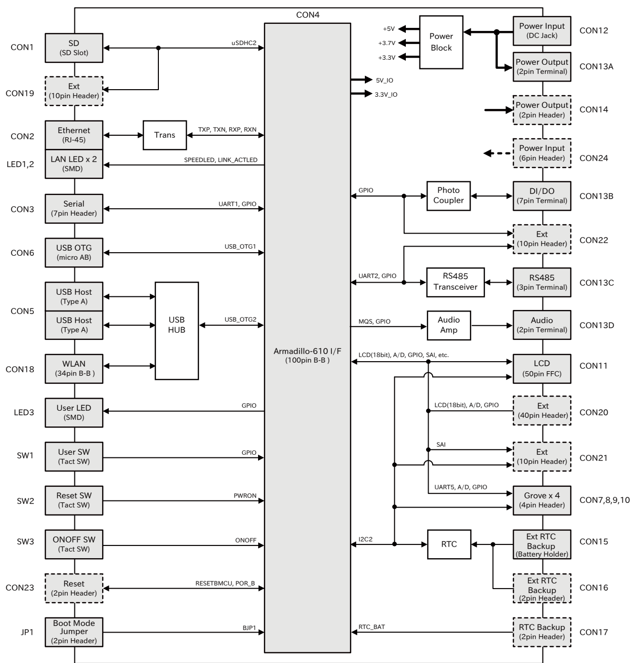
図 6.182 Armadillo-610 拡張ボードのブロック図
