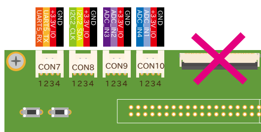
図 6.192 Armadillo-610 拡張ボード CON7、CON8、CON9、CON10
