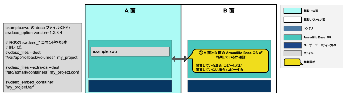
図 6.79 Armadillo Base OS を B 面にコピー
