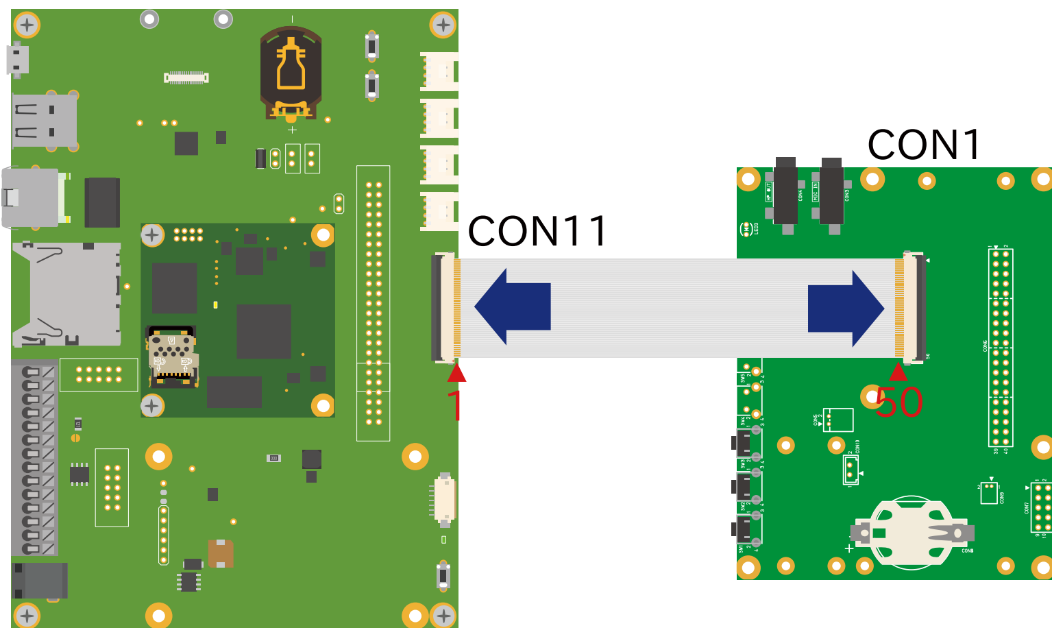
図 6.224 Armadillo-610 と LCD 拡張ボードの接続
