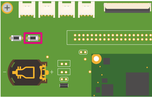
図 6.215 Armadillo-610 拡張ボード SW3
