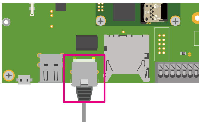
図 6.186 Armadillo-610 拡張ボード CON2
