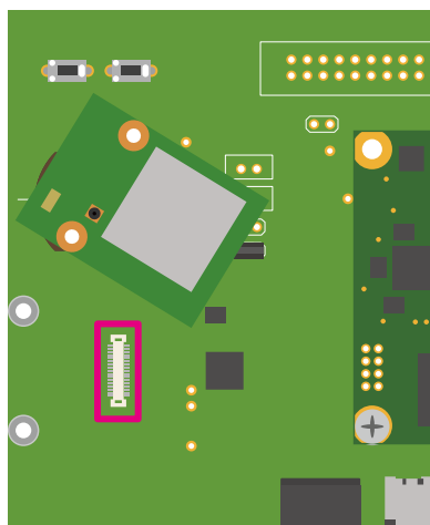
図 6.205 Armadillo-610 拡張ボード CON18
