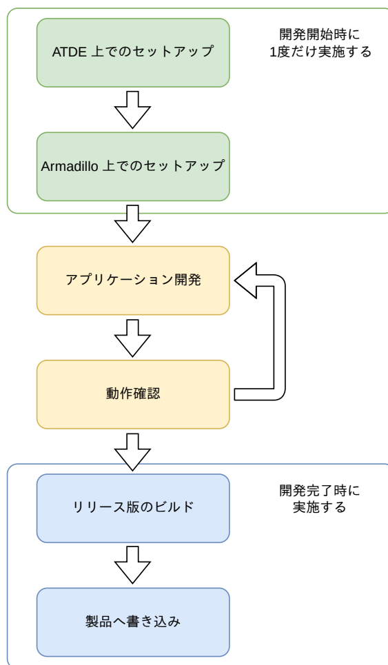
図 3.210 C 言語によるアプリケーション開発の流れ
