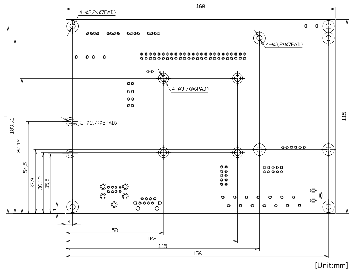
図 6.218 Armadillo-610 拡張ボード 基板形状および固定穴寸法
