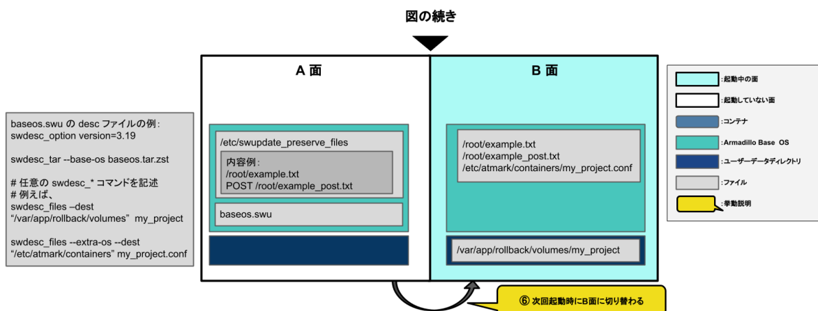
図 6.86 B 面への切り替え (component=base_os)
