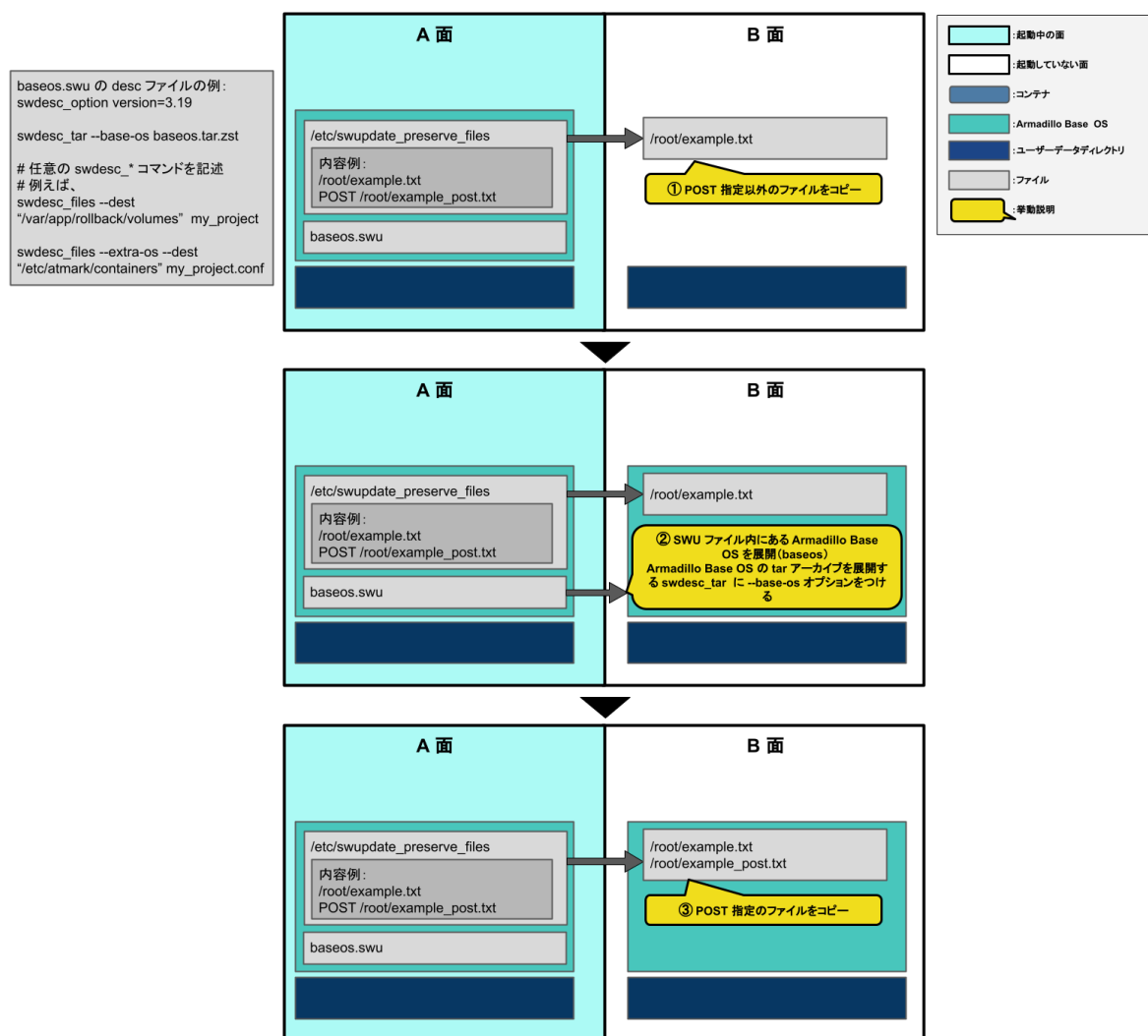
図 6.83 Armadillo Base OS とファイルを B 面にコピー
