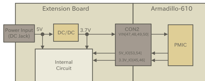
図 3.60 電源回路例
