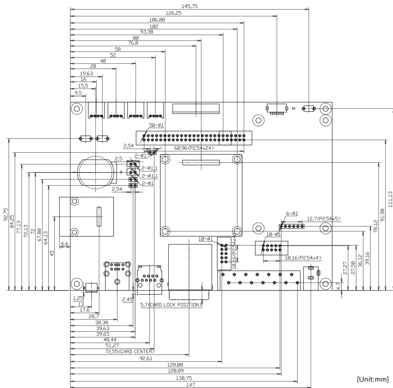
図 6.219 Armadillo-610 拡張ボード コネクタ中心寸法および穴寸法
