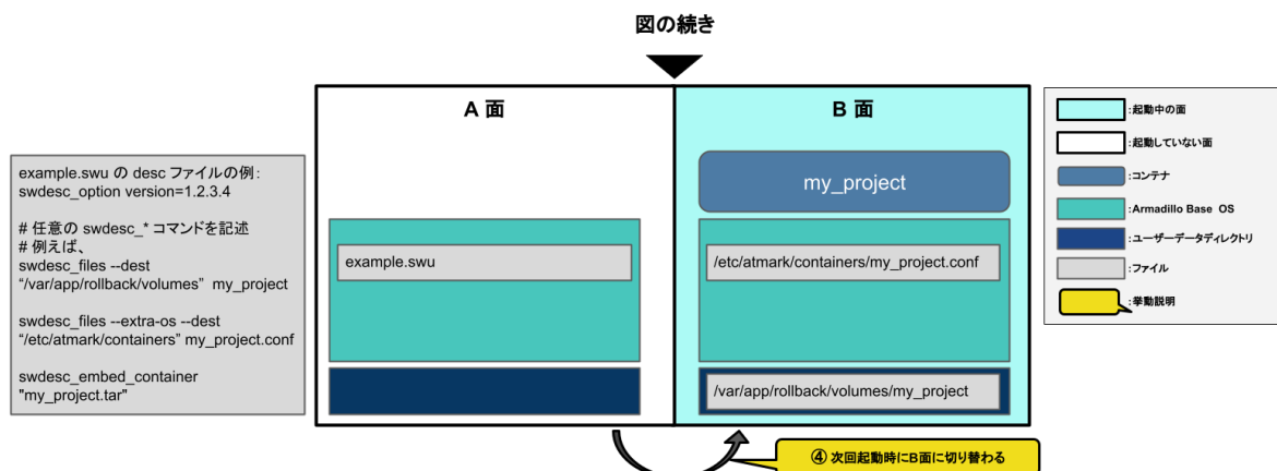
図 6.82 B 面への切り替え
