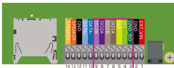
図 6.197 CON13B の配置
