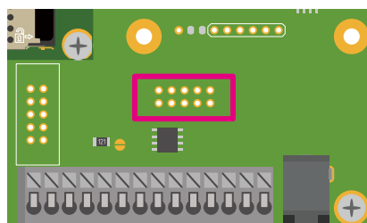
図 6.209 Armadillo-610 拡張ボード CON22
