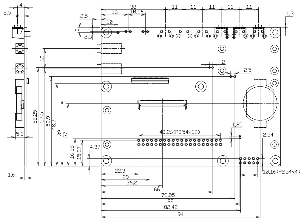
図 6.228 LCD 拡張ボードのコネクタ位置寸法
