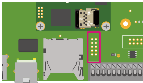
図 6.206 Armadillo-610 拡張ボード CON19
