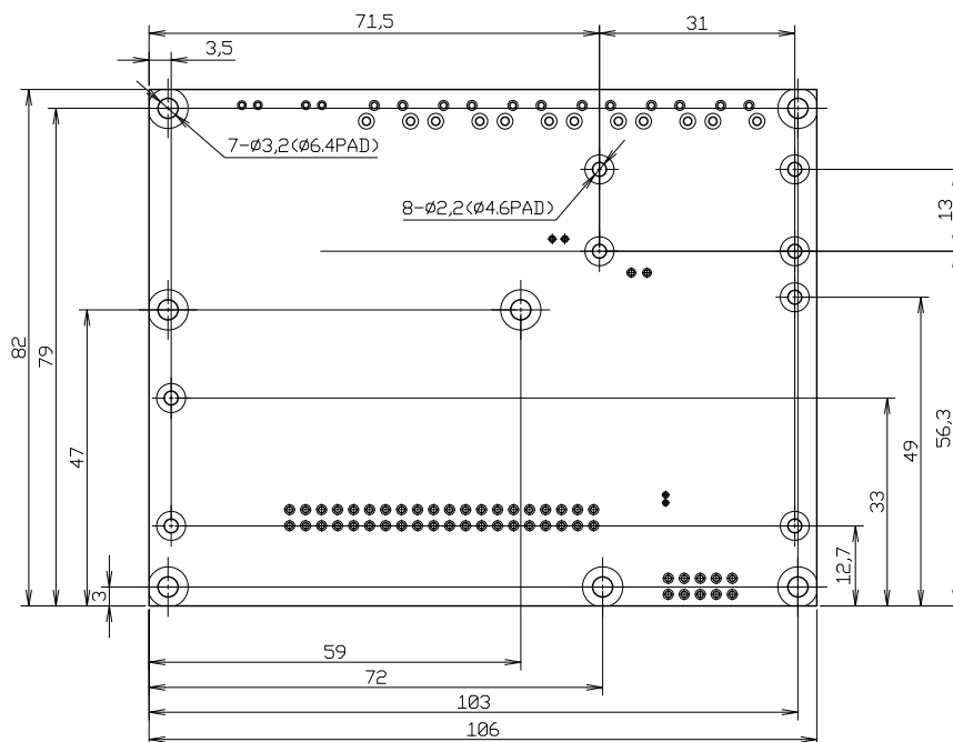
図 6.226 LCD 拡張ボードの基板形状および固定穴寸法
