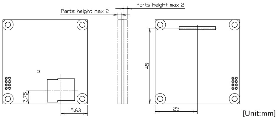
図 3.81 コネクタ中心寸法
