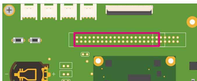
図 6.200 Armadillo-610 拡張ボード CON20
