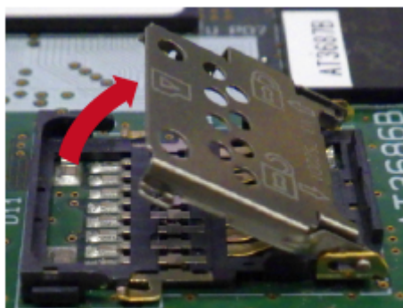
図 3.99 カバーを開ける
