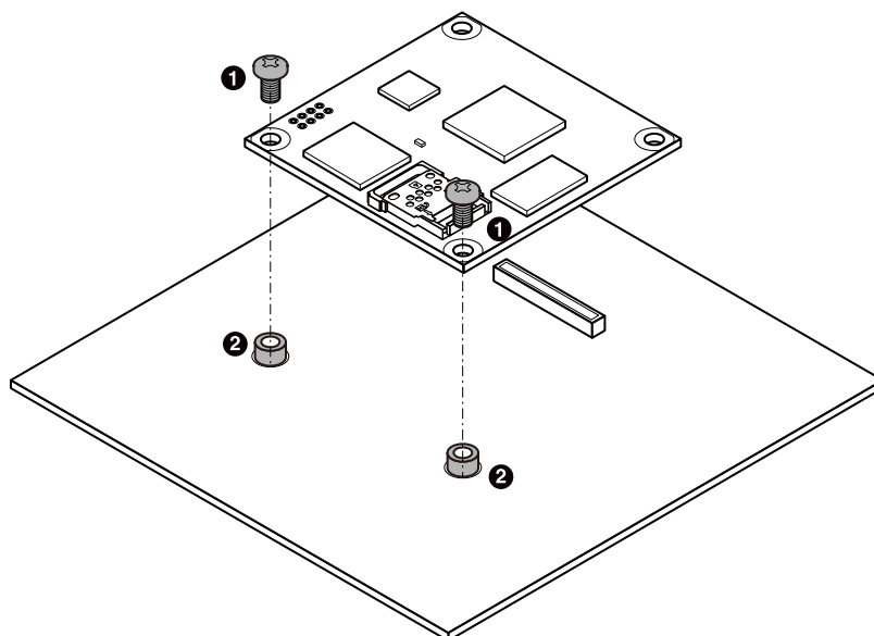
図 3.74 Armadillo-610 の固定例
