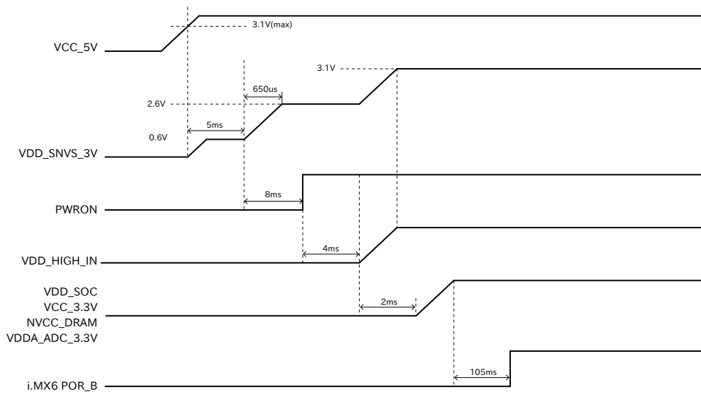
図 3.76 電源シーケンス [6]
