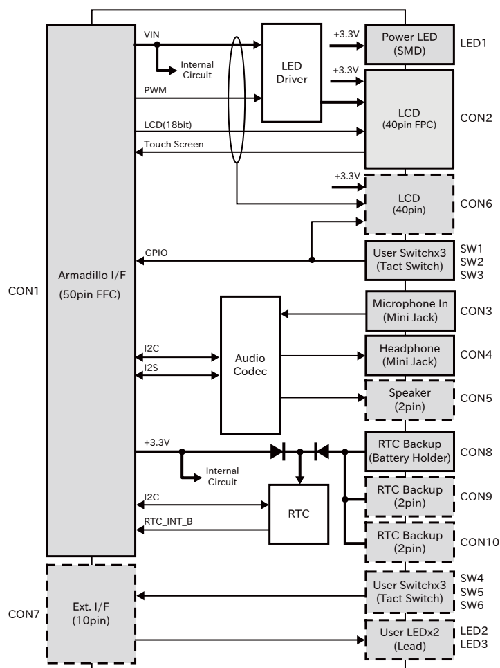
図 6.213 LCD 拡張ボードのブロック図
