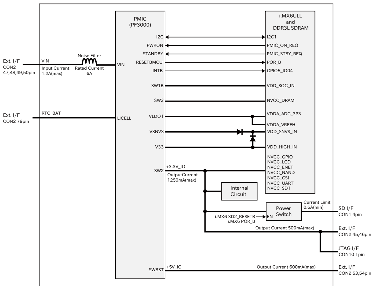
図 3.75 電源回路の構成
