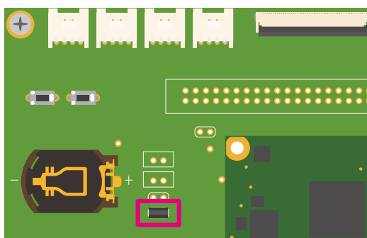
図 6.205 Armadillo-610 拡張ボード JP1
