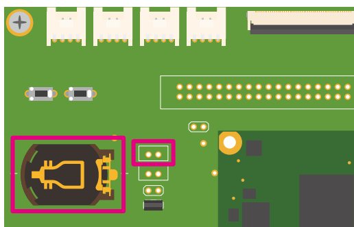
図 6.195 Armadillo-610 拡張ボード CON15、CON16
