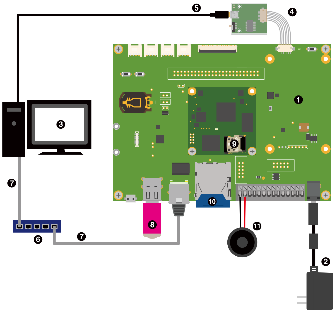
図 3.58 Armadillo-610 開発セットの接続例
