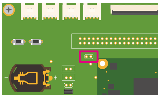
図 6.194 Armadillo-610 拡張ボード CON14
