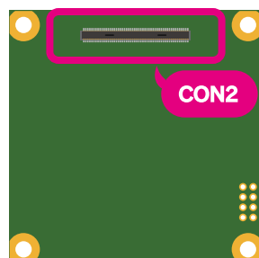
図 3.60 Armadillo-610 の CON2
