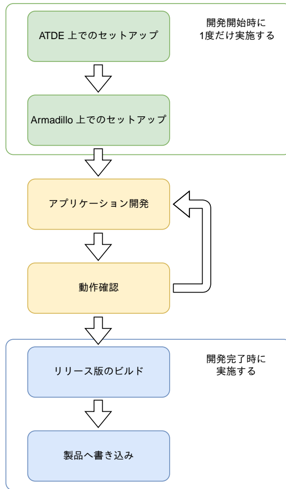
図 3.202 C 言語によるアプリケーション開発の流れ
