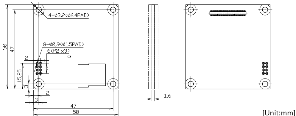
図 3.80 基板形状および固定穴寸法
