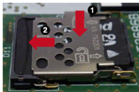
図 3.103 カバーをロックする
