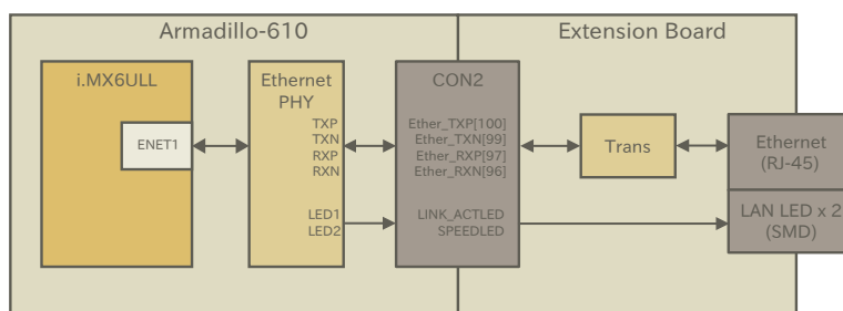
図 3.64 LAN(Ethernet)接続例
