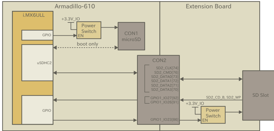
図 3.68 SD 接続例
