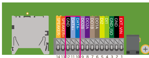
図 6.138 CON13C の配置
