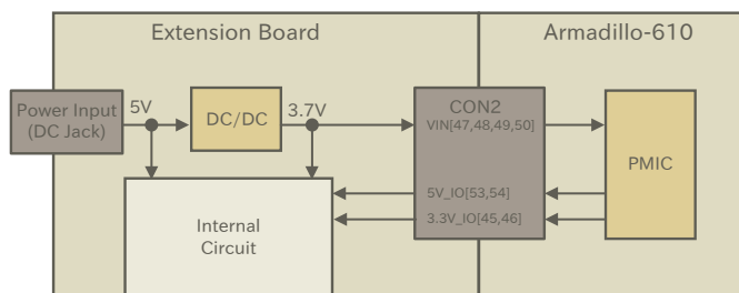
図 3.29 電源回路例
