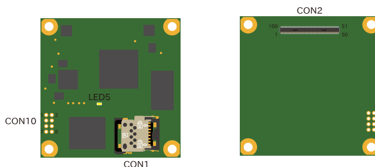
図 2.6 Armadillo-610 インターフェースレイアウト
