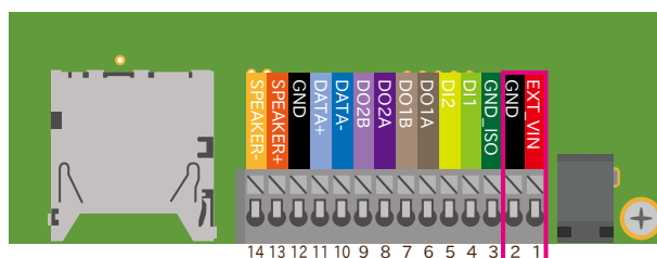
図 6.136 CON13A の配置
