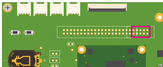
図 6.147 Armadillo-610 拡張ボード CON21
