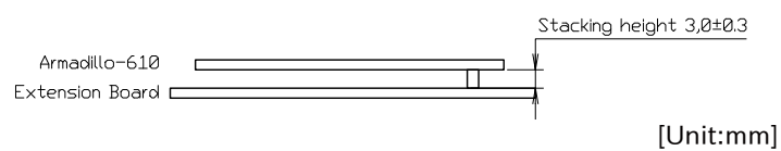
図 3.49 Armadillo-610 のスタッキング高さ
