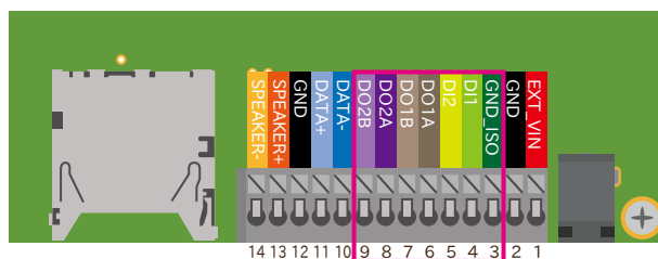
図 6.137 CON13B の配置
