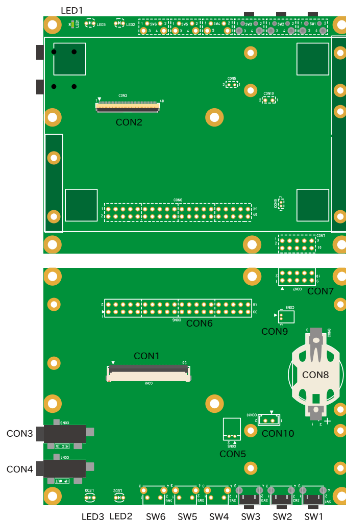
図 6.160 LCD 拡張ボードのインターフェース
