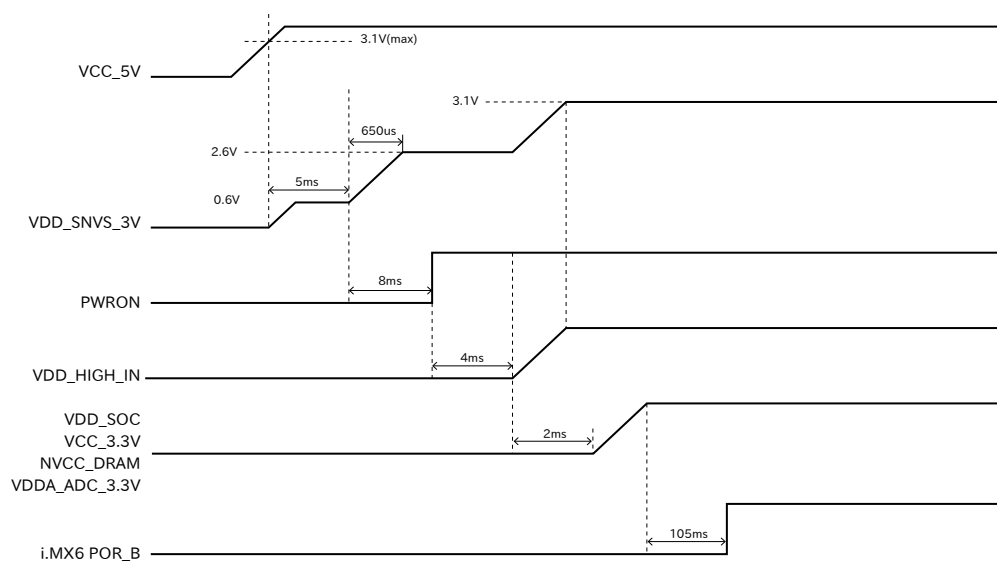
図 3.43 電源シーケンス [6]
