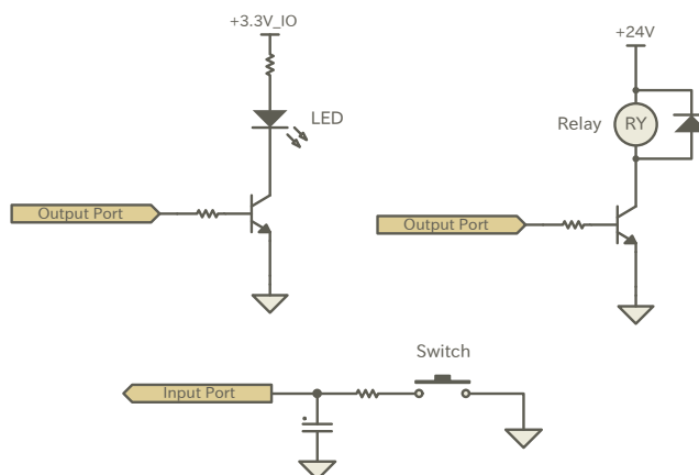
図 3.36 スイッチ、LED、リレー接続例
