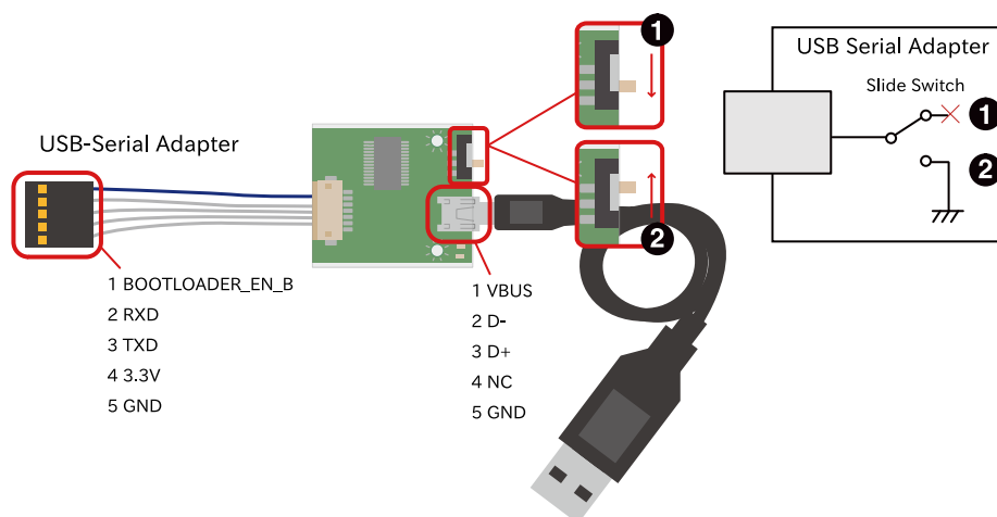
図 6.121 USB シリアル変換アダプタの配線
