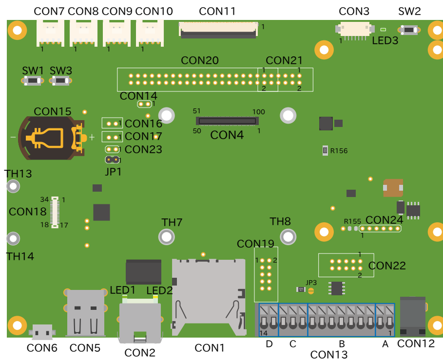
図 2.7 Armadillo-610 拡張ボード インターフェースレイアウト
