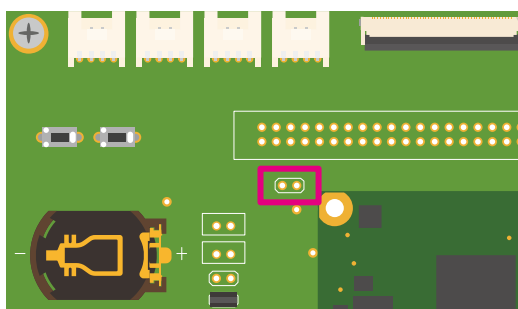
図 6.140 Armadillo-610 拡張ボード CON14
