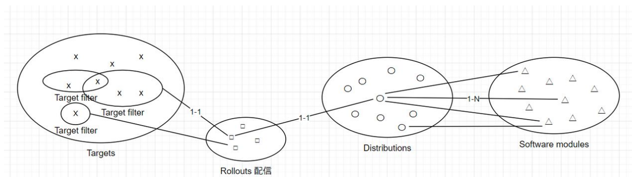
図 5.9 hawkBit が扱うソフトウェアのデータ構造
