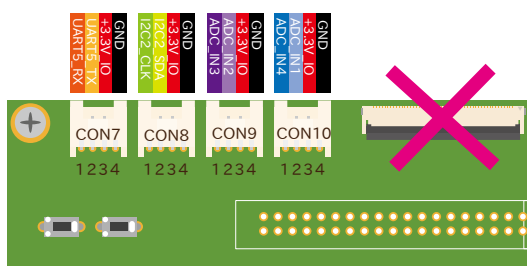
図 6.132 Armadillo-610 拡張ボード CON7、CON8、CON9、CON10
