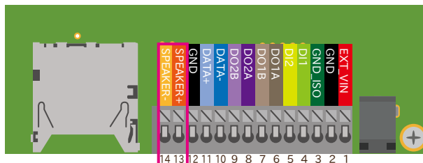
図 6.147 CON13D の配置
