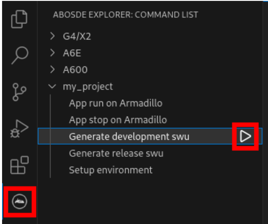
図 3.137 リリース版をビルドする
