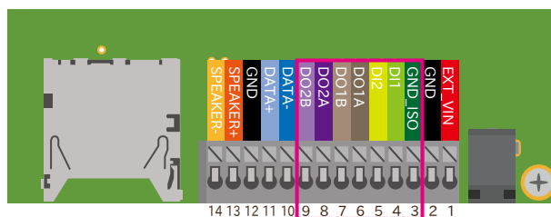
図 6.145 CON13B の配置
