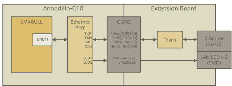
図 3.34 LAN(Ethernet)接続例
