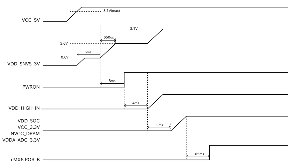
図 6.122 電源シーケンス [2]
