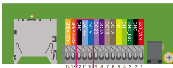
図 6.146 CON13C の配置
