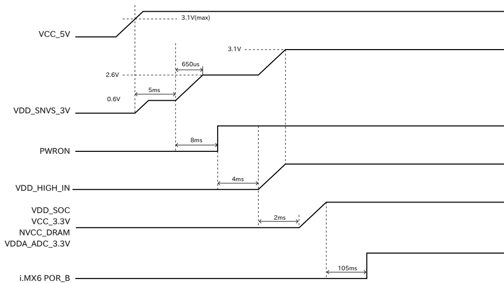
図 6.122 電源シーケンス [2]
