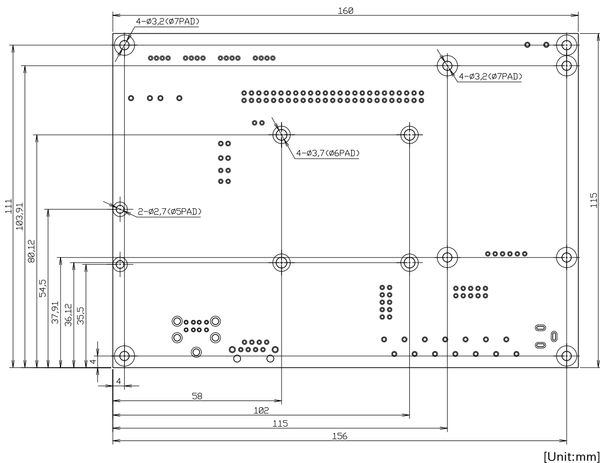
図 6.165 Armadillo-610 拡張ボード 基板形状および固定穴寸法
