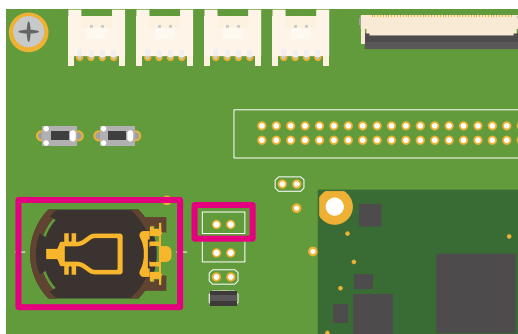
図 6.149 Armadillo-610 拡張ボード CON15、CON16
