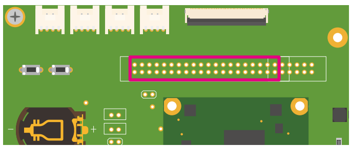
図 6.154 Armadillo-610 拡張ボード CON20
