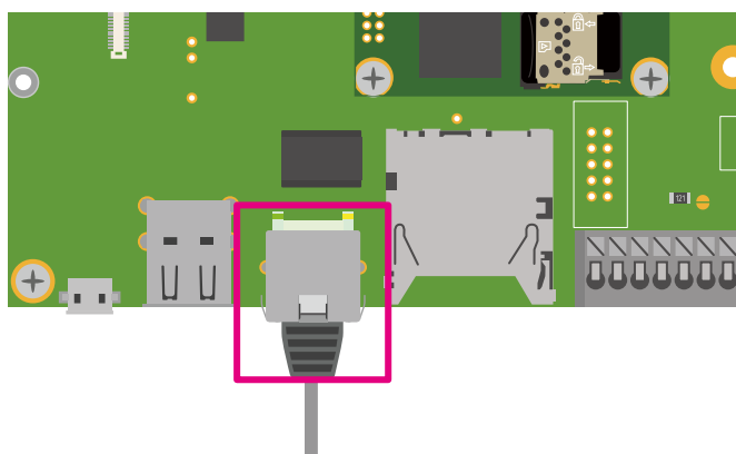
図 6.134 Armadillo-610 拡張ボード CON2
