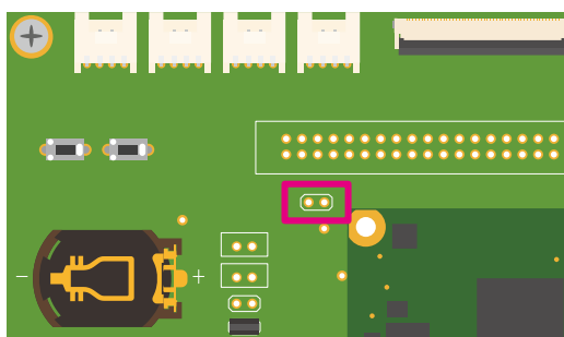
図 6.148 Armadillo-610 拡張ボード CON14
