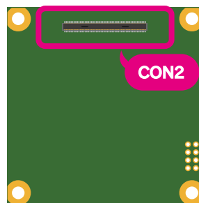
図 3.30 Armadillo-610 の CON2
