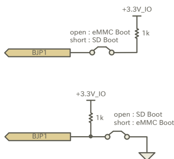
図 3.33 起動設定ジャンパー例
