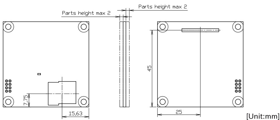
図 6.127 コネクタ中心寸法
