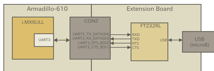
図 3.37 シリアル(UART)接続例
