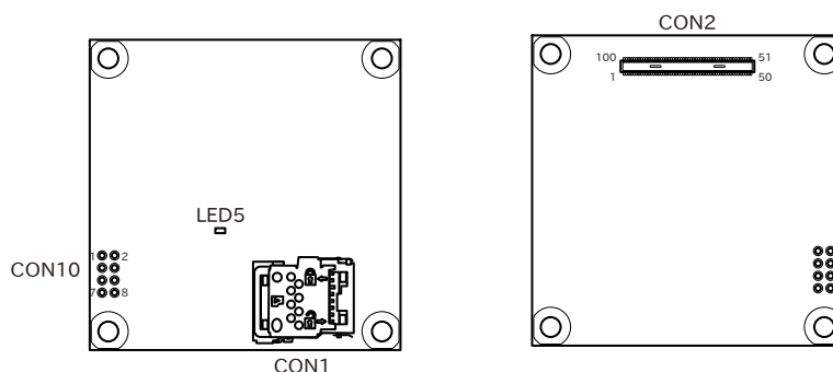
図 3.59 Armadillo-610 のインターフェース
