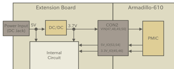
図 3.32 電源回路例
