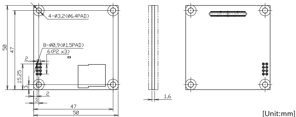
図 6.126 基板形状および固定穴寸法
