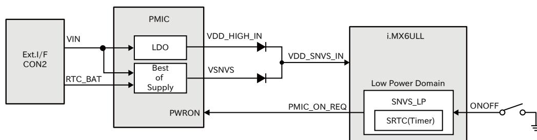
図 6.125 ONOFF 回路の構成 [3]
