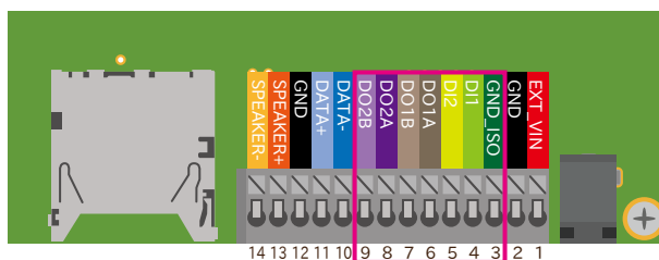
図 6.145 CON13B の配置
