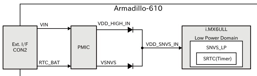
図 6.151 バックアップ電源供給回路
