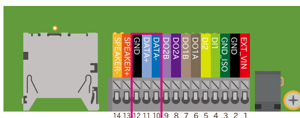
図 6.146 CON13C の配置
