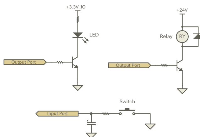
図 14.25 スイッチ、LED、リレー接続例
