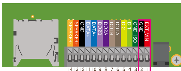
図 15.16 CON13A の配置
