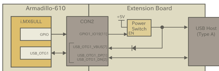
図 14.22 USB Host 接続例
