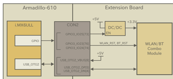
図 14.21 WLAN/BT 接続例
