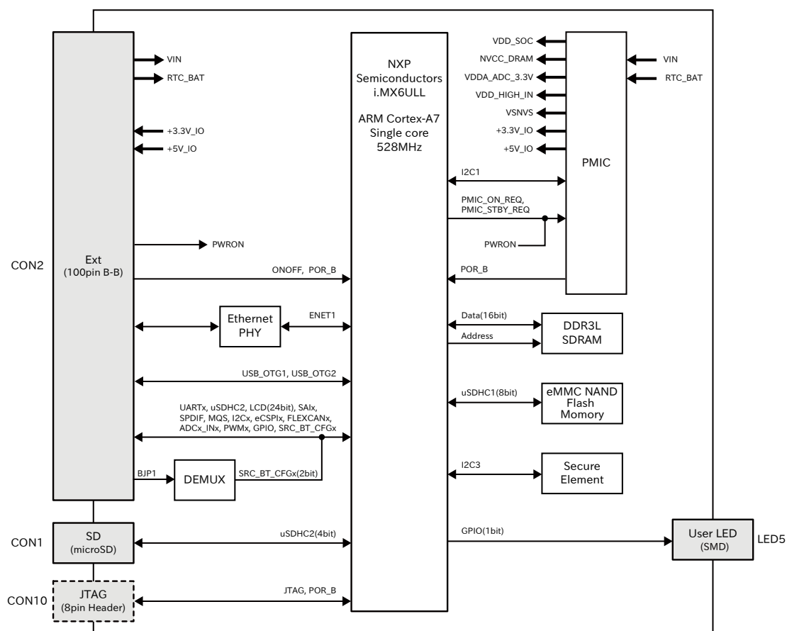
図 3.6 Armadillo-610 ブロック図
