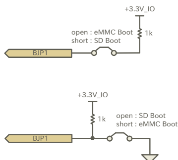
図 14.19 起動設定ジャンパー例
