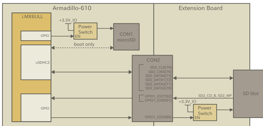
図 14.24 SD 接続例
