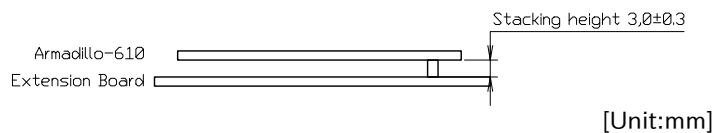
図 14.15 Armadillo-610 のスタッキング高さ
