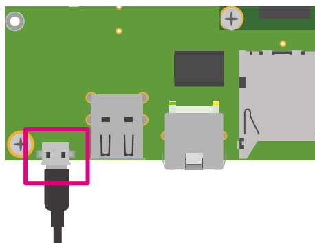
図 15.11 Armadillo-610 拡張ボード CON6
