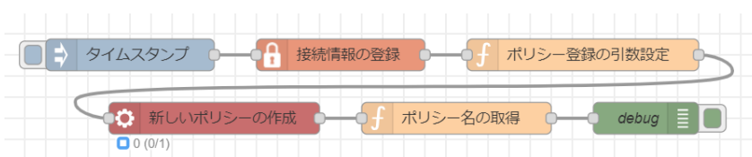
図 4.47 ポリシーを作成するフロー
