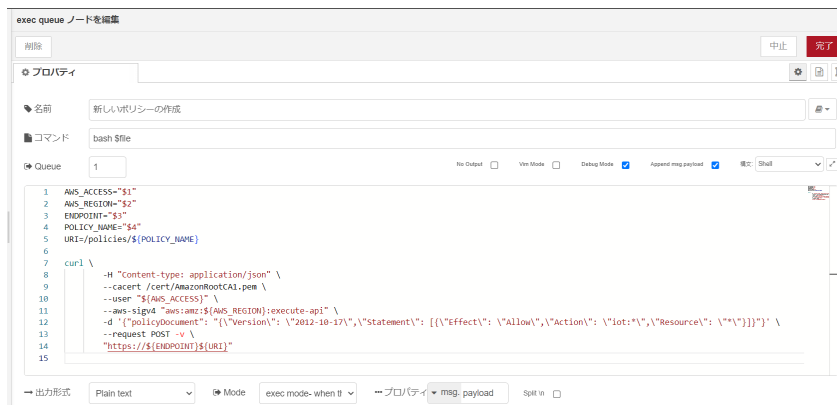
図 4.45 [新しいポリシーの作成] ノードのプロパティ内容
