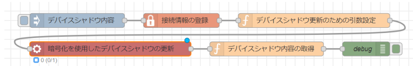
図 4.69 データの暗号化を使用したデバイスシャドウを更新するフロー
