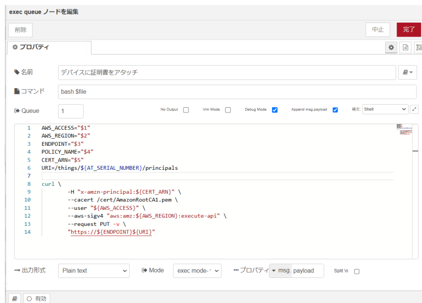
図 4.57 [証明書をデバイスにアタッチ] ノードのプロパティ内容
