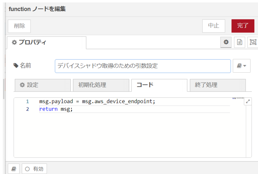
図 4.60 [デバイスシャドウ取得のための引数設定] ノードのプロパティ内容
