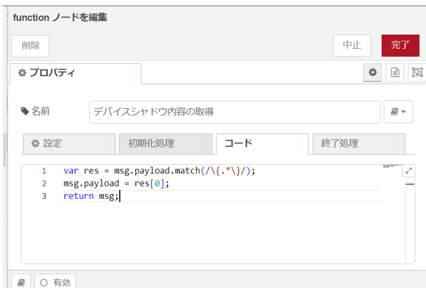
図 4.68 [デバイスシャドウ内容の取得] ノードのプロパティ内容
