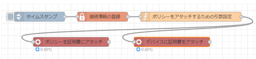
図 4.58 デバイスにポリシーをアタッチするフロー
