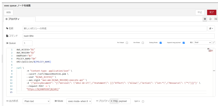
図 4.45 [新しいポリシーの作成] ノードのプロパティ内容
