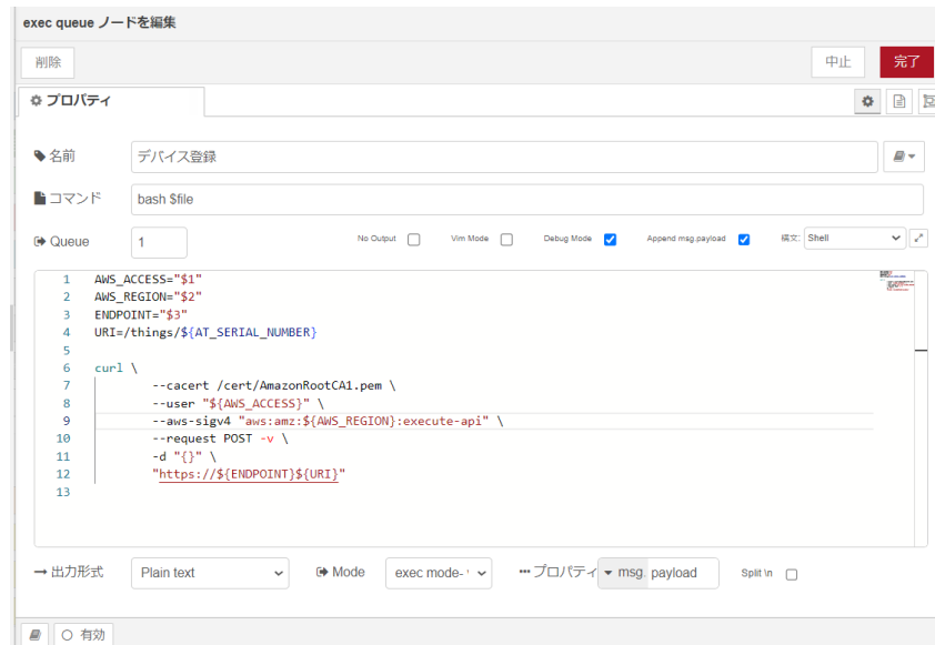
図 4.39 [exec queue] ノードのプロパティ内容
