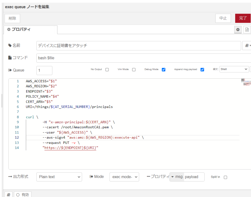
図 4.57 [証明書をデバイスにアタッチ] ノードのプロパティ内容
