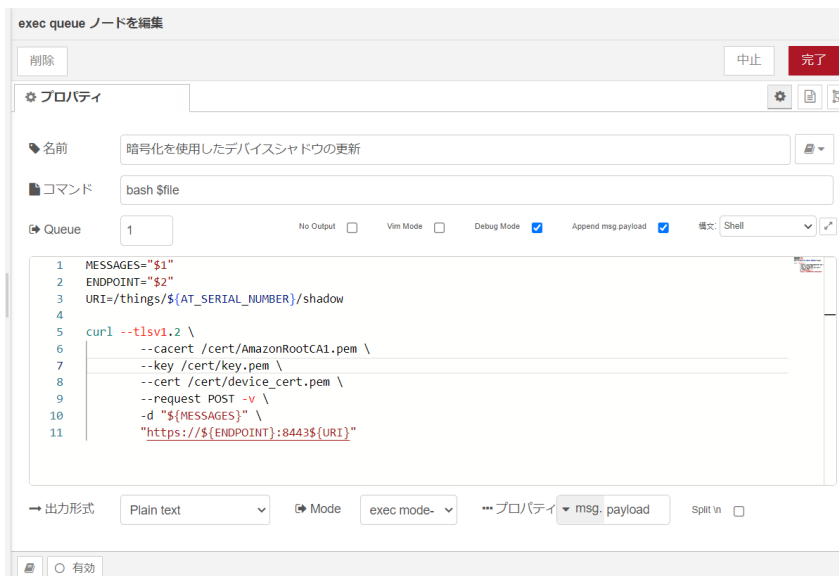
図 4.67 [暗号化を使用したデバイスシャドウの更新] ノードのプロパティ内容
