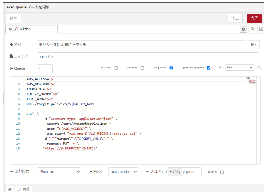
図 4.56 [ポリシーを証明書にアタッチ] ノードのプロパティ内容
