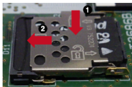
図 5.21 カバーをロックする
