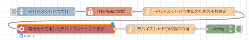
図 4.69 データの暗号化を使用したデバイスシャドウを更新するフロー
