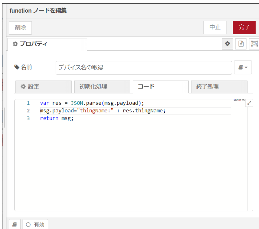
図 4.40 [デバイス名の取得] ノードのプロパティ内容
