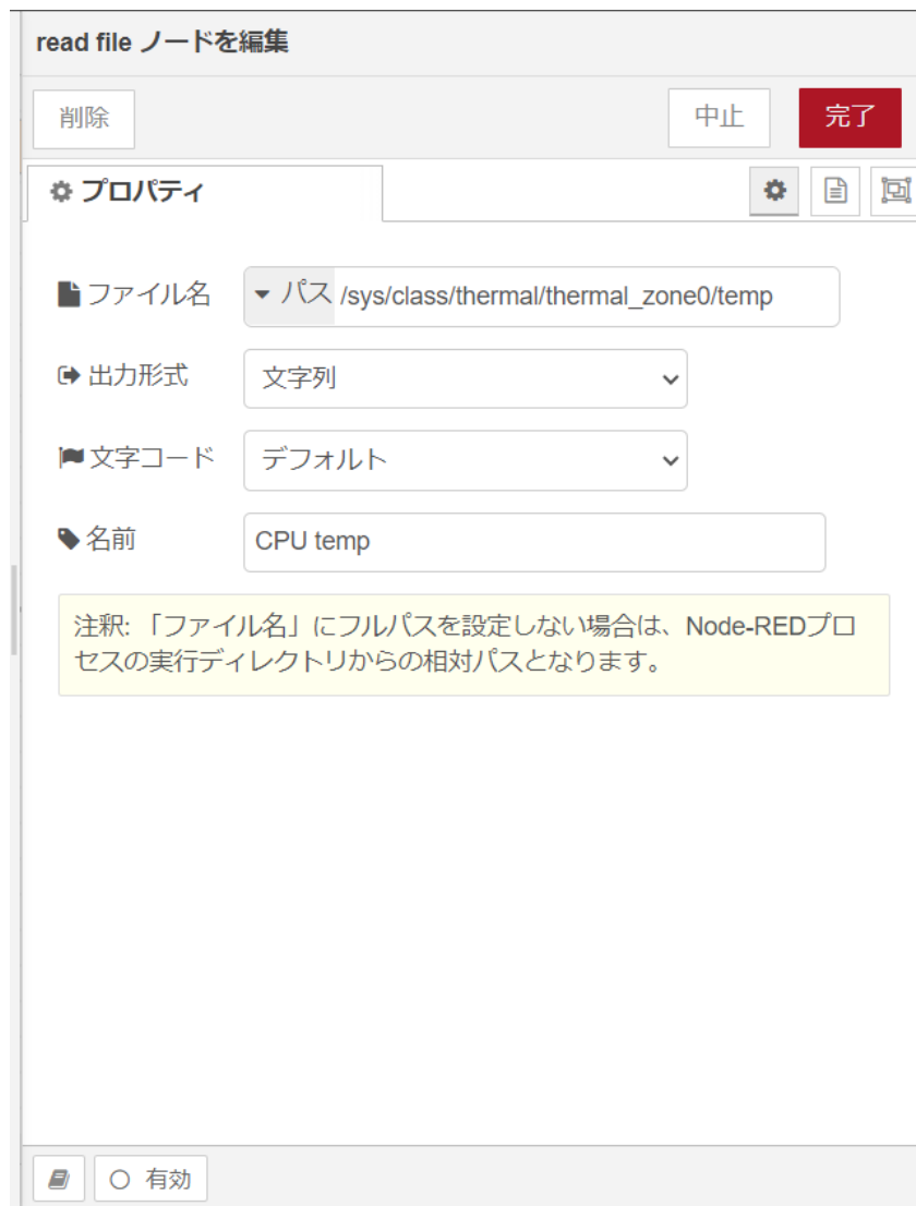
図 4.9 [read file] ノードのプロパティ内容
