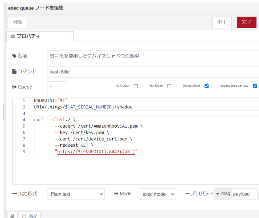
図 4.61 [暗号化を使用したデバイスシャドウの取得] ノードのプロパティ内容
