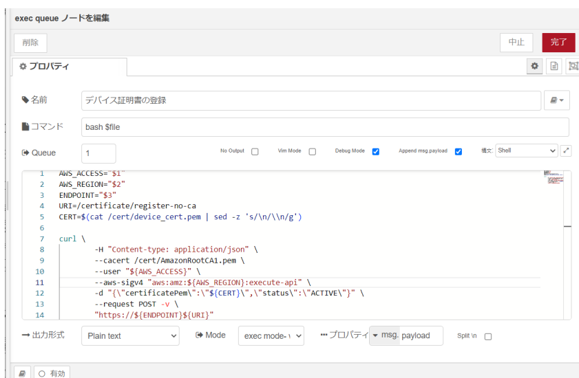
図 4.50 [デバイス証明書の登録] ノードのプロパティ内容
