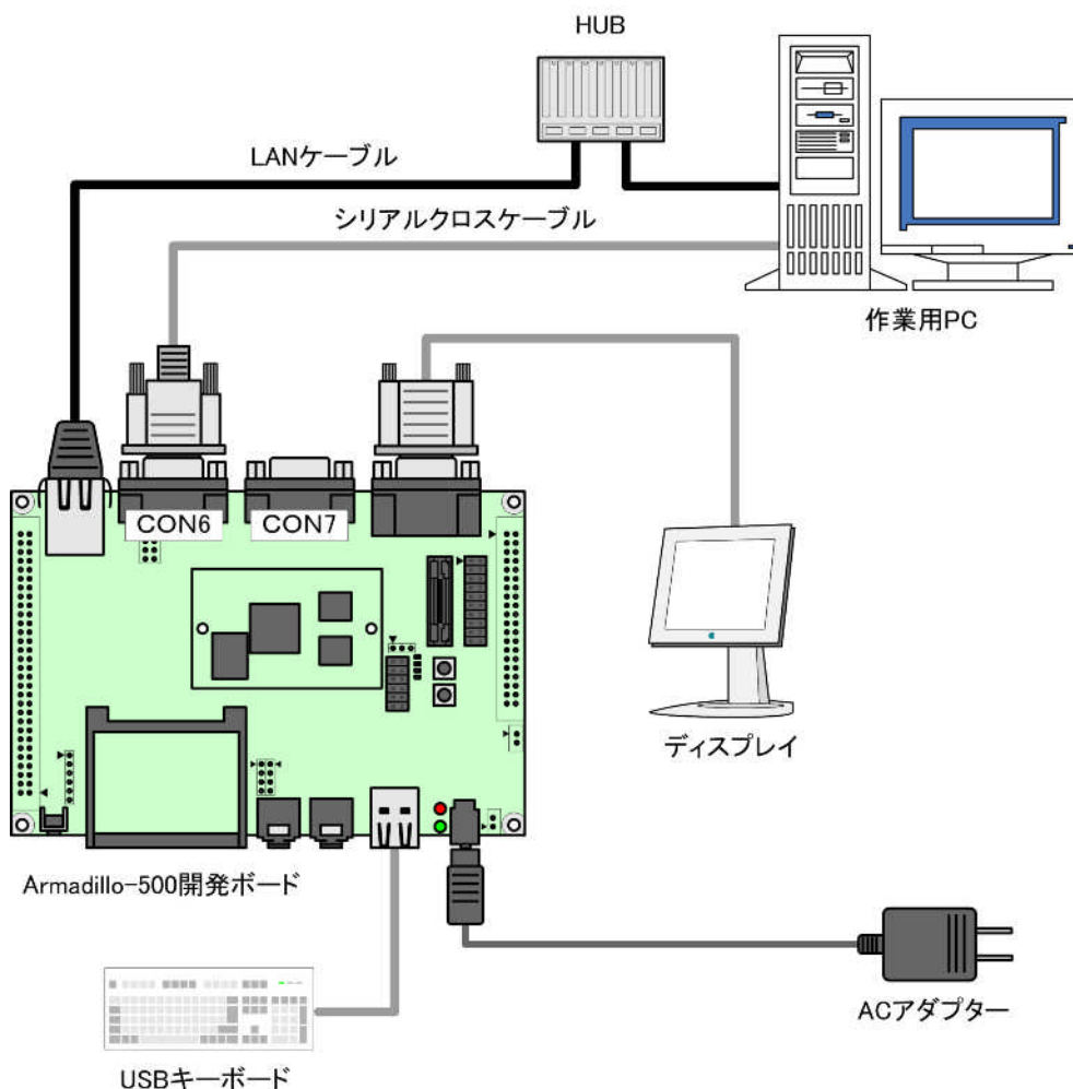
図 2.2. 接続図
