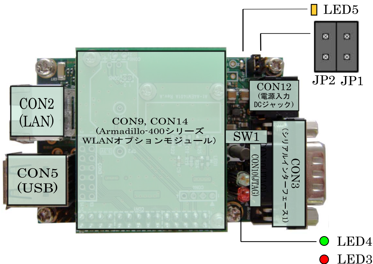
図 3.5 Armadillo-420 WLAN モデル(AWL13 対応)見取り図
