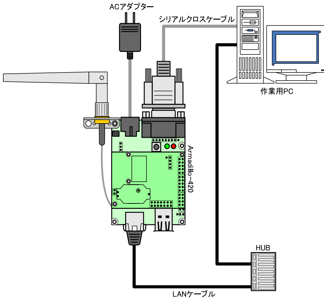
図 4.3 Armadillo-420 WLAN モデル(AWL13 対応)接続例
