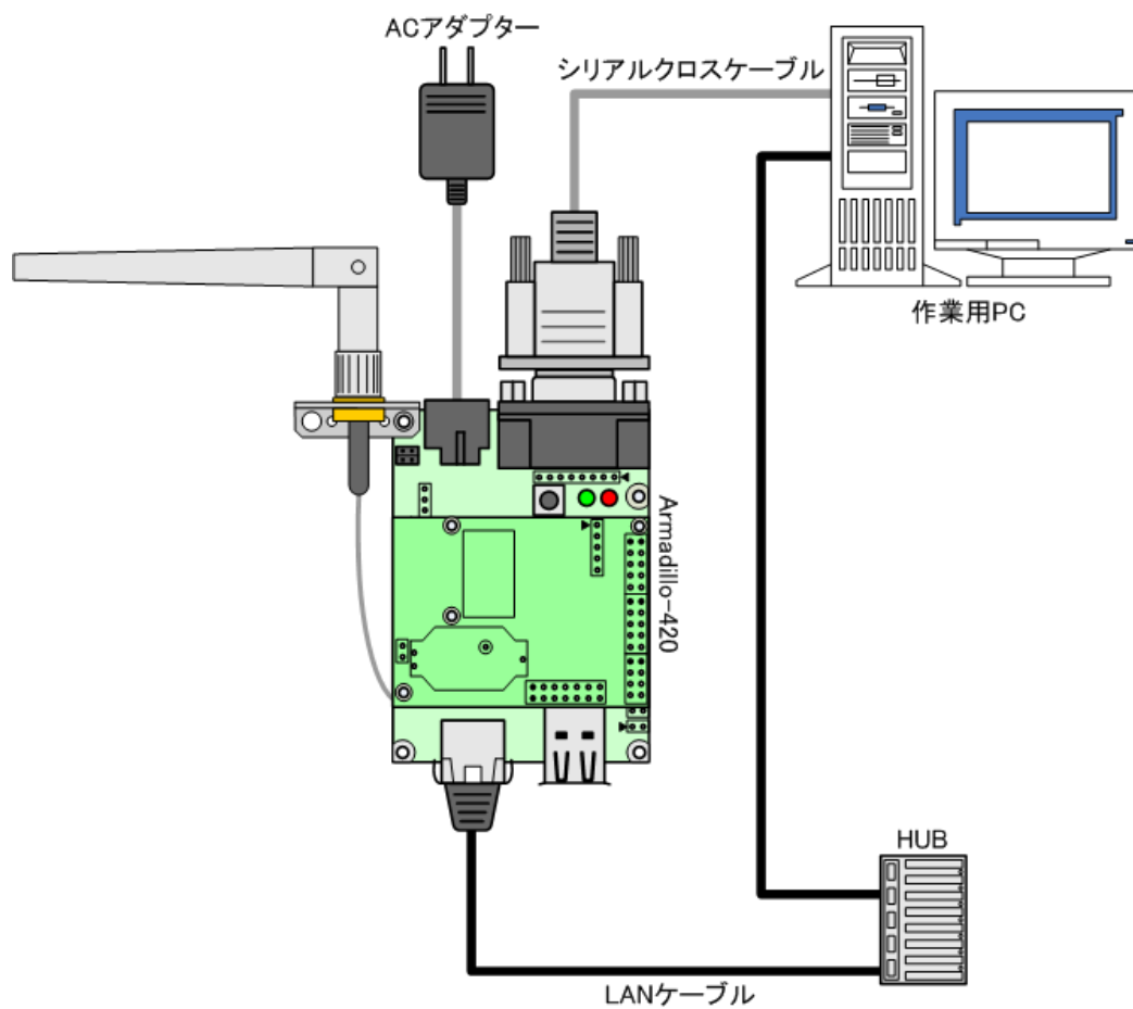
図 4.2 Armadillo-420 WLAN モデル(AWL12 対応)接続例
