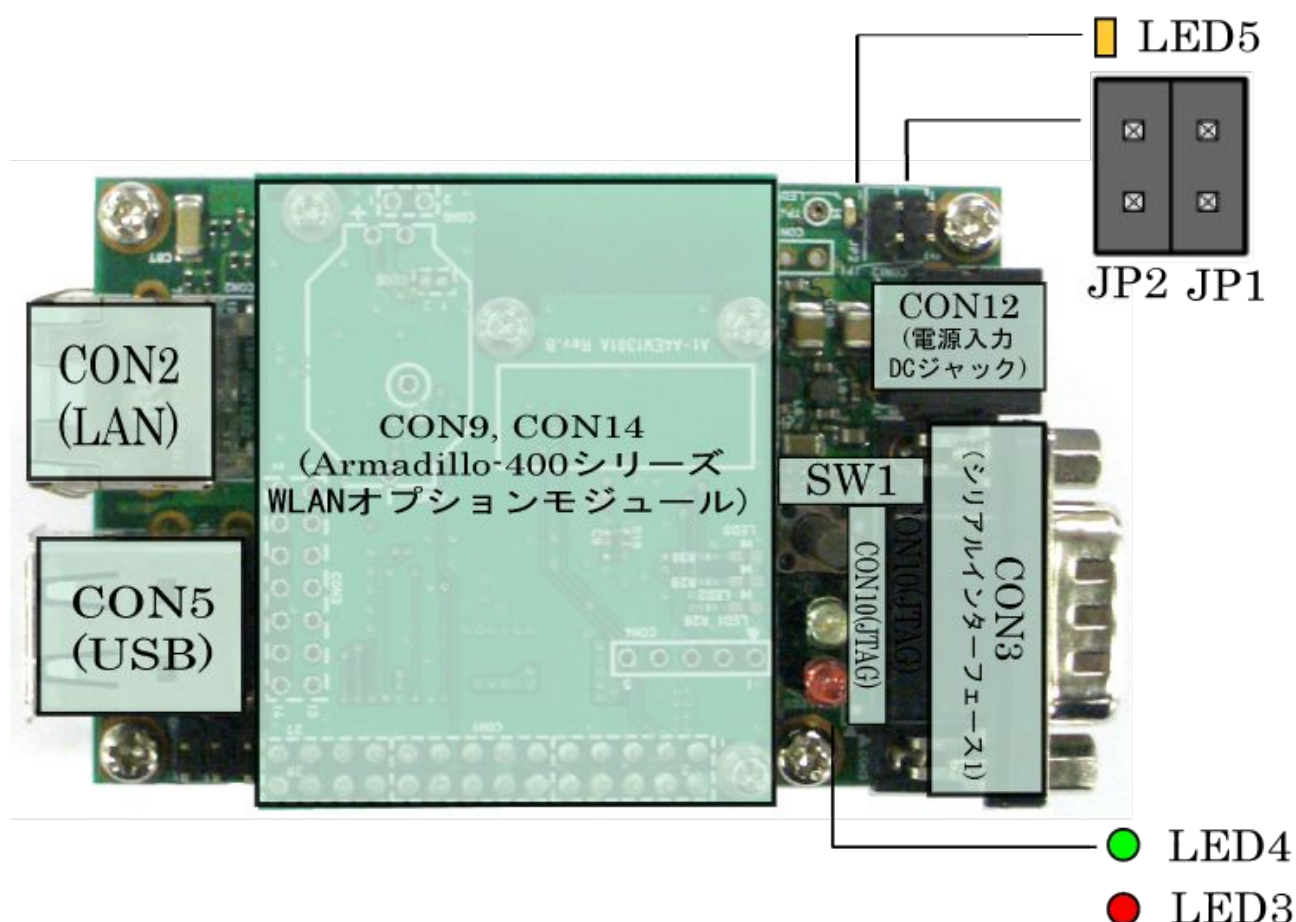
図 3.4 Armadillo-420 WLAN モデル(AWL12 対応)見取り図
