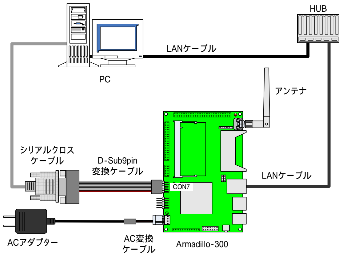
図 3-1 接続図
