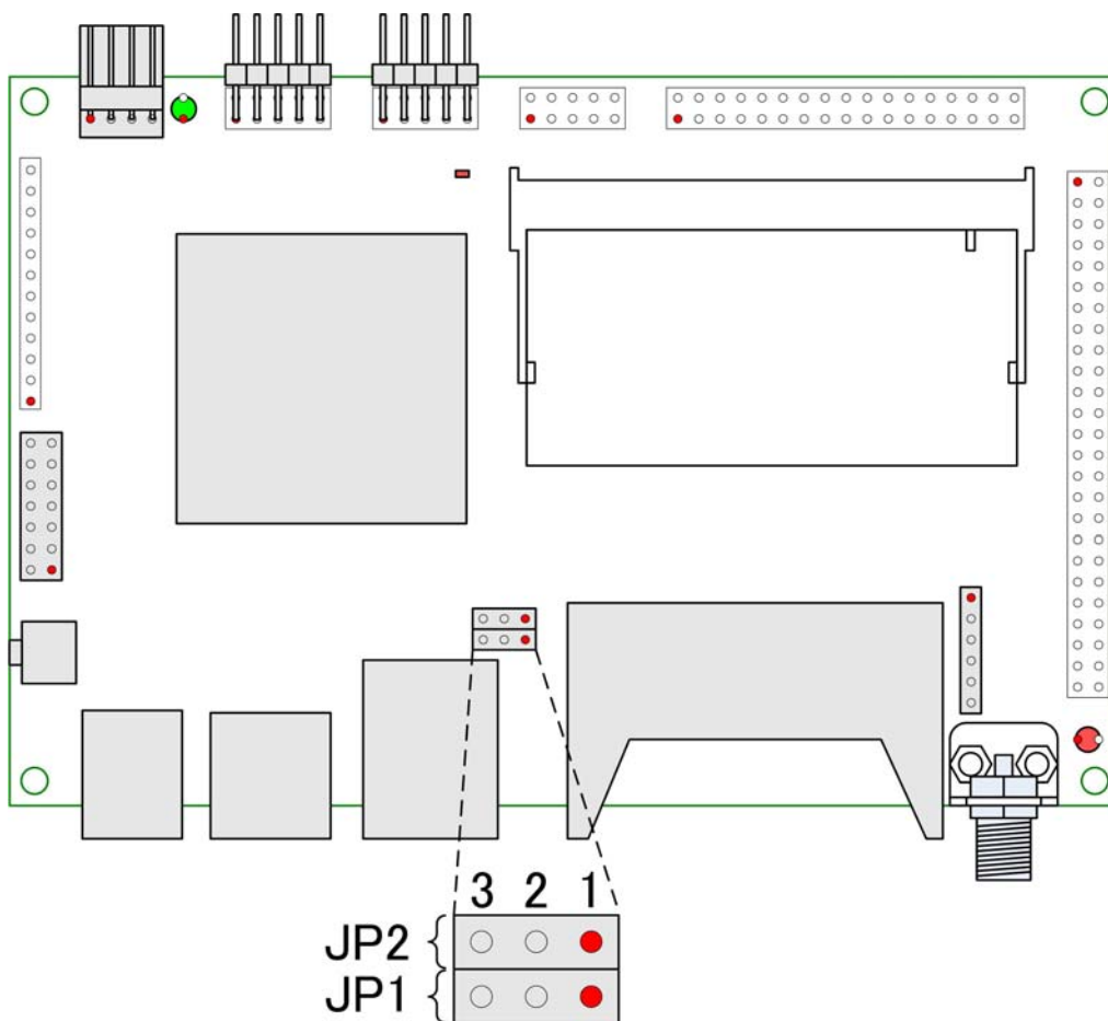
図 3-2 ジャンパピンの位置
