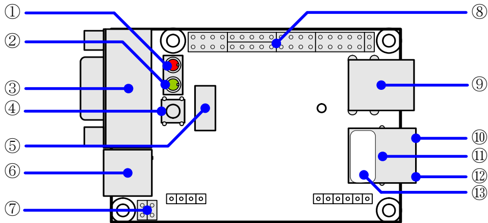
図 3-1 Armadillo-240 のインターフェース
