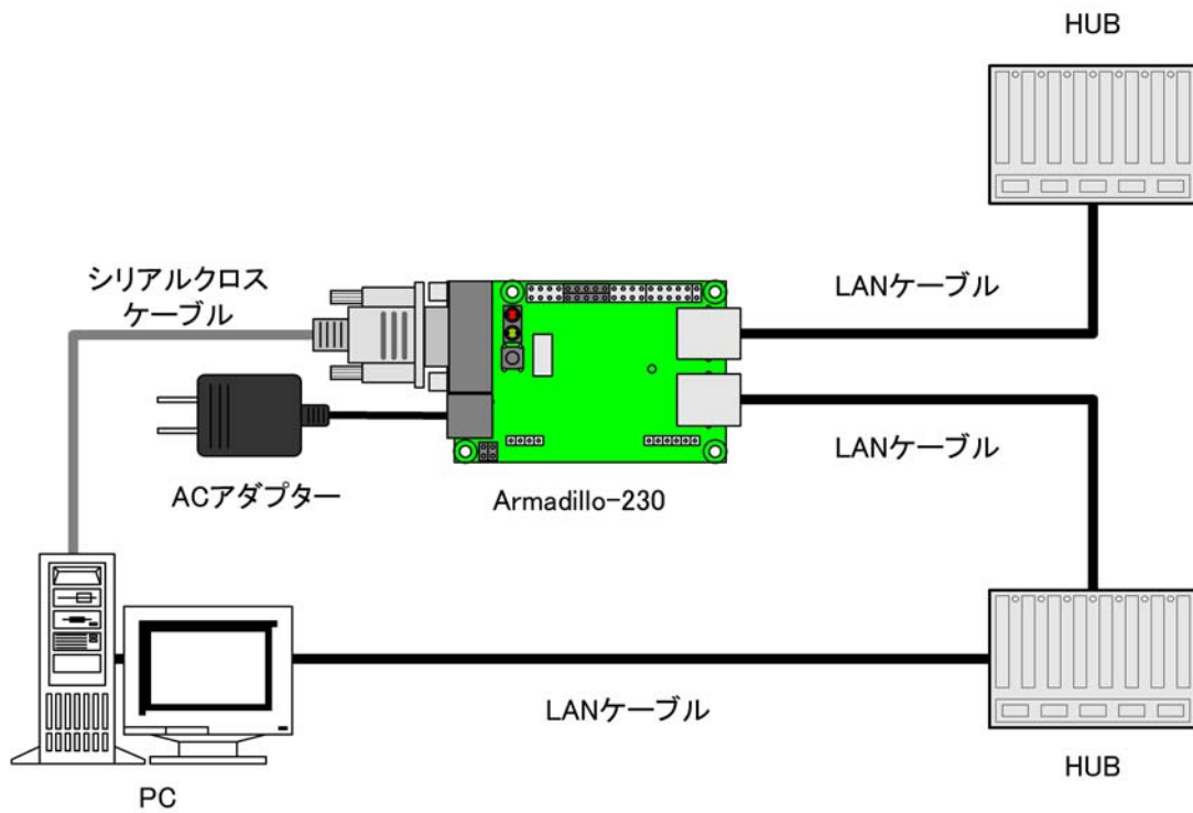
図 2-2 Armadillo-230 接続例
