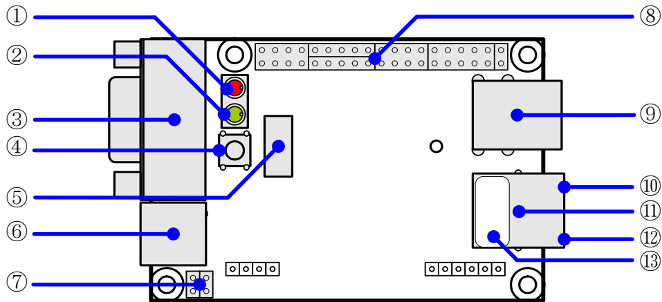
図 3-1 Armadillo-220 のインターフェース
