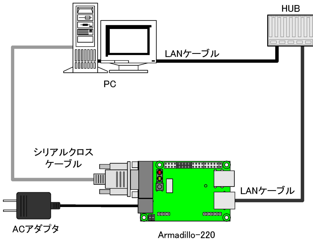
図 2-1 Armadillo-220 接続例
