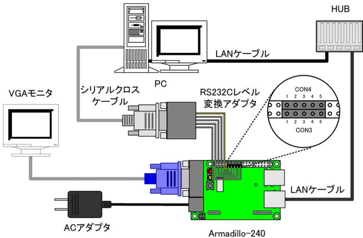
図 2-3 Armadillo-240 接続例
