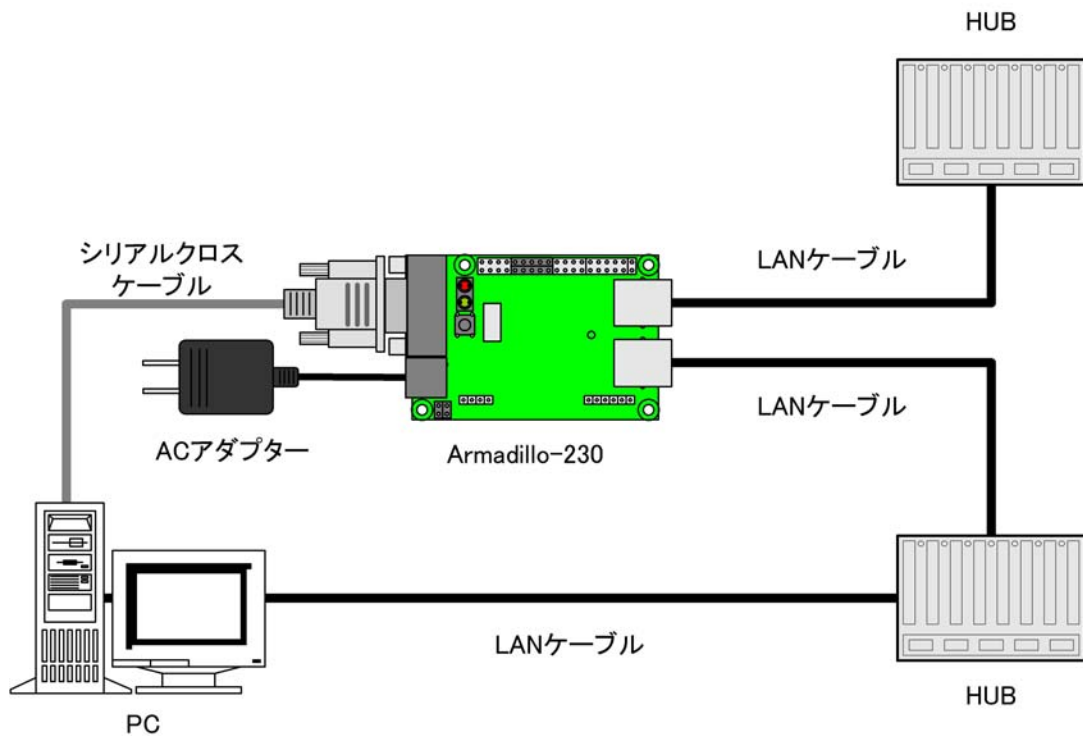
図 2-2 Armadillo-230 接続例
