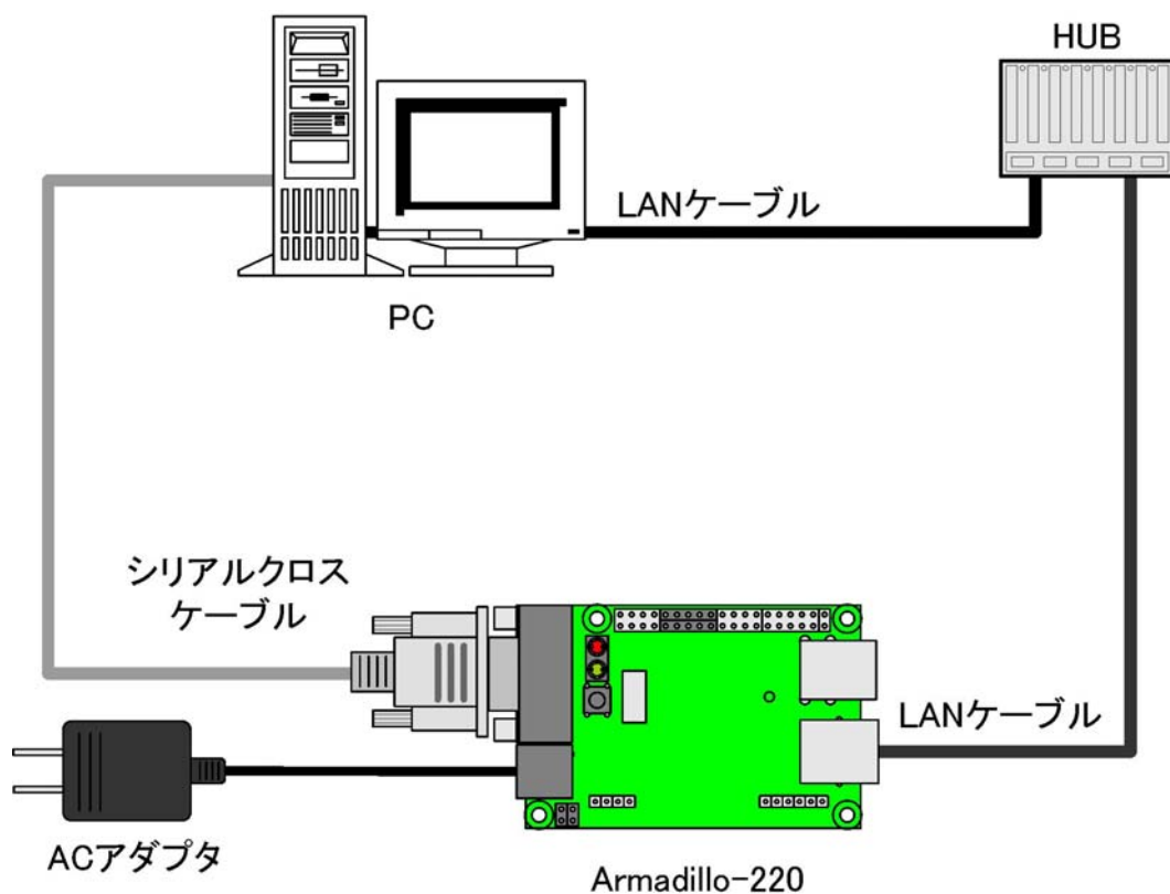
図 2-1 Armadillo-220 接続例
