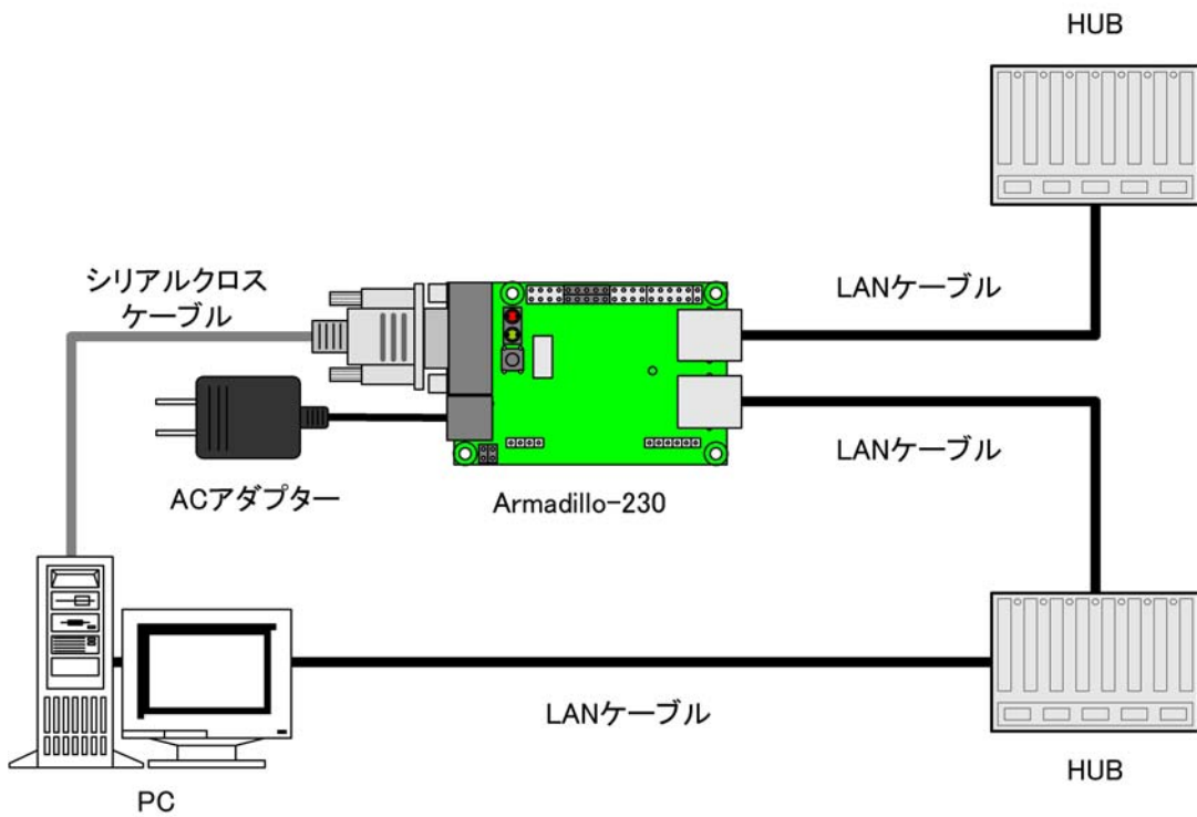
図 2-2 Armadillo-230 接続例
