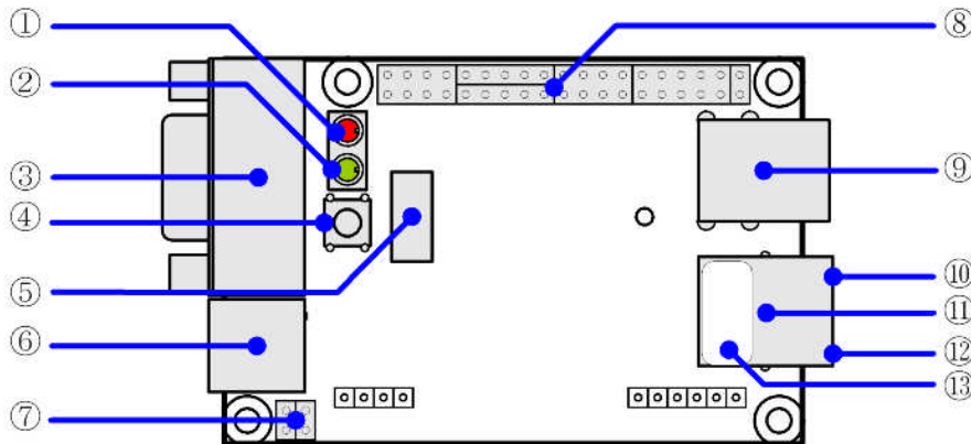
図 3.1. Armadillo-220 のインターフェース
