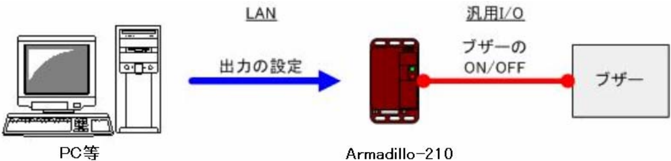
図 6-2 ブザー(出力ポート)の出力を設定する場合
