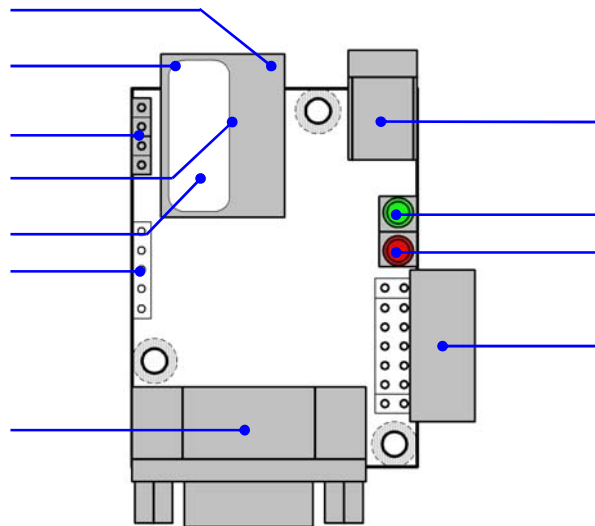
図 3-1 Armadillo-210 のインターフェース
