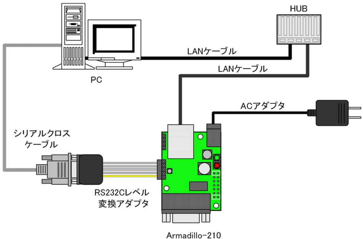
図 2-1 Armadillo-210 接続例
