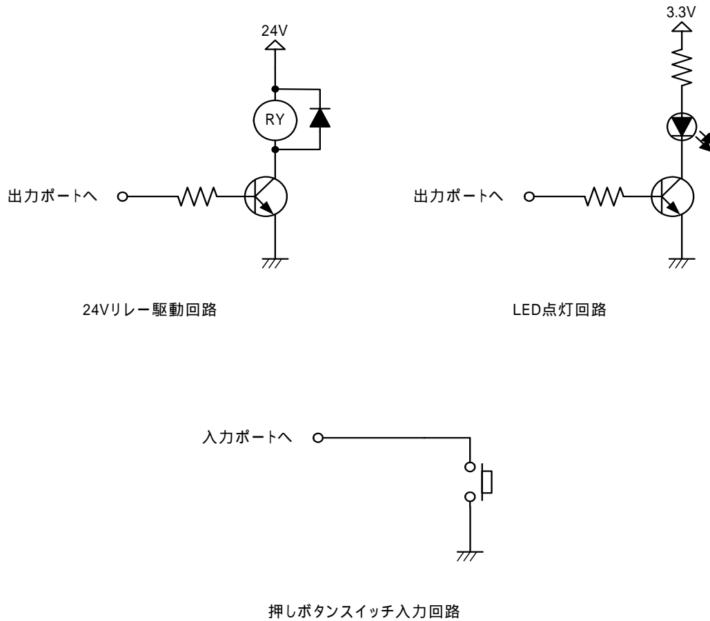
図 6-1 参考回路例
