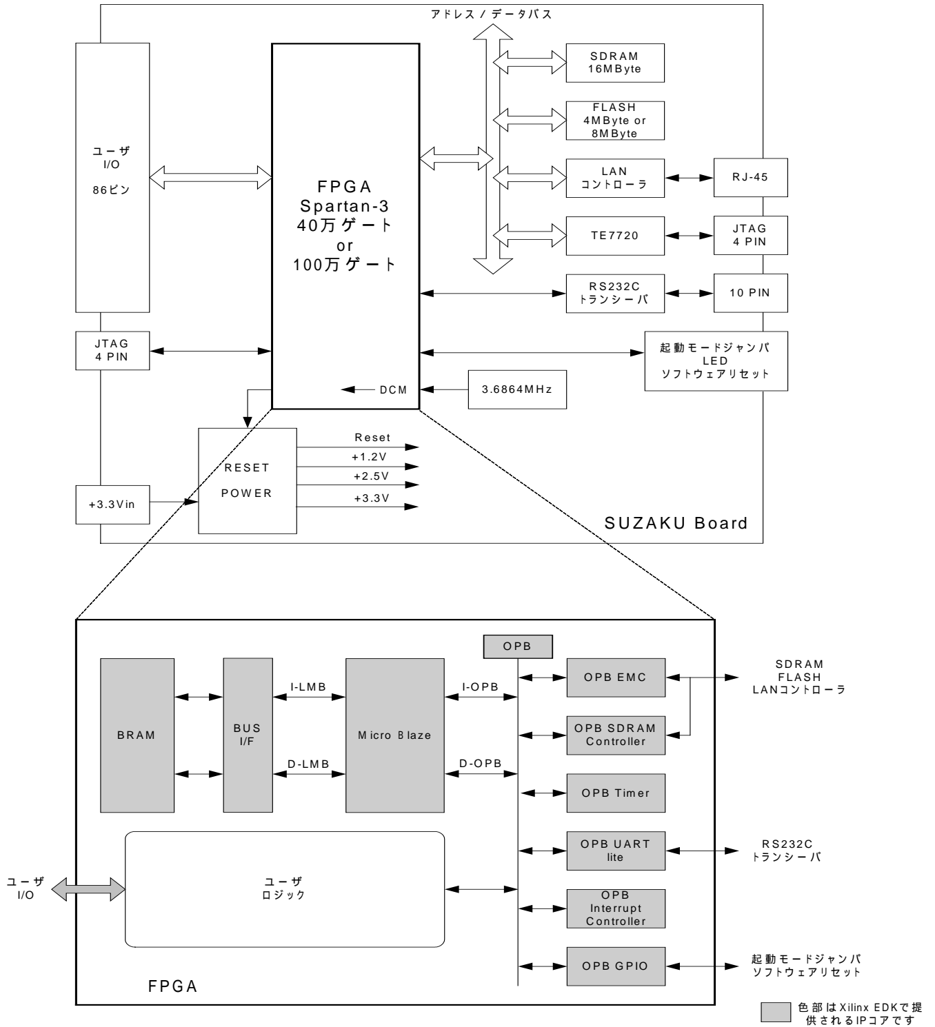
図 4-1 SUZAKU ブロック図
