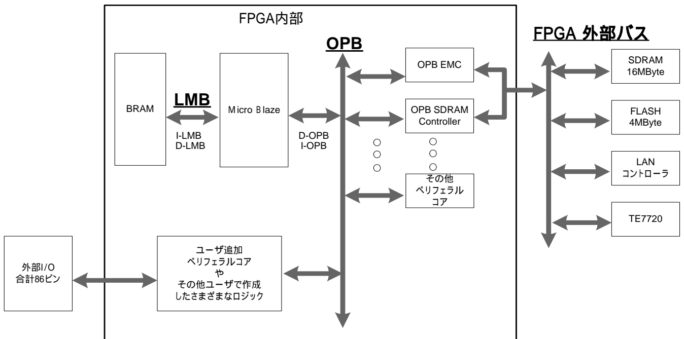
図 4-2 SUZAKU バス構成
