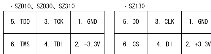
図 8-2 Flash書き込み ピンアサイン
